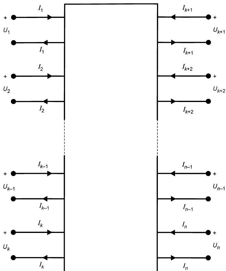
Рисунок 2 — Обозначения, используемые в линейных n -полюсниках
