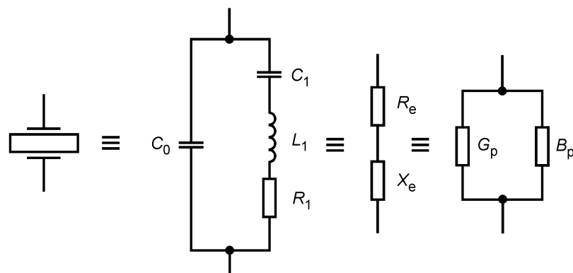
Рисунок 3 — Эквивалентные схемы пьезоэлектрического резонатора (см. элементы 1101, 1102, 1003, 1104 и 1106)
