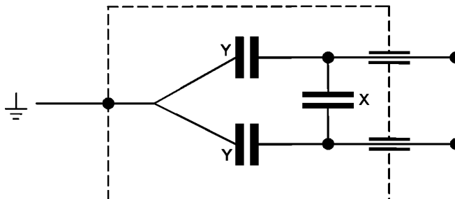
Рисунок 5b — Соединение развязывающих конденсаторов треугольником (в металлическом корпусе)
