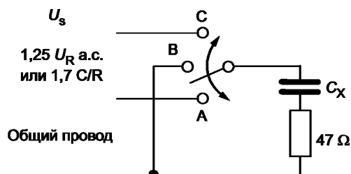
Рисунок В.1 — Цепь для испытания на долговечность
