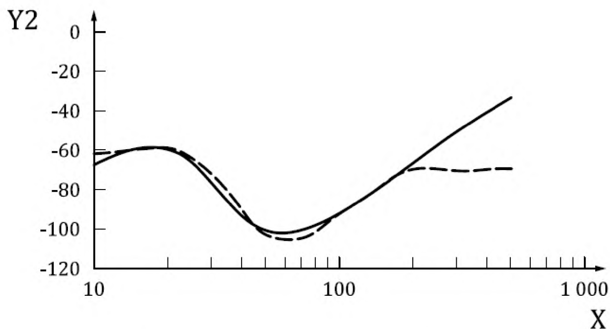
Рисунок В.4 — Сравнение результатов моделирования (сплошная линия) и опорных значений (пунктирная линия) эффективной массы системы «кисть — рука» в направлении z_h
