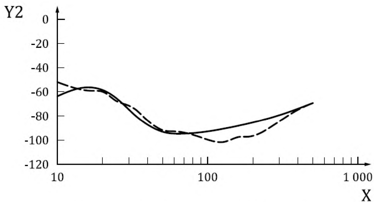
Рисунок В.3 — Сравнение результатов моделирования (сплошная линия) и опорных значений (пунктирная линия) эффективной массы системы «кисть — рука» в направлении y_h
