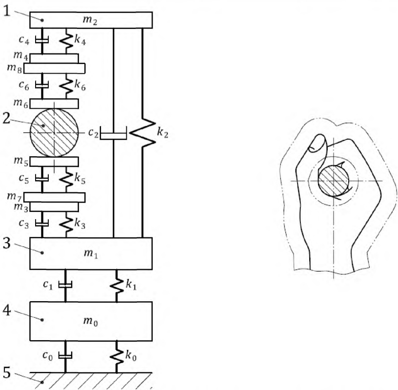
1 — пальцы; 2 — рукоятка; 3 — ладонь, запястье и предплечье; 4 — верхняя часть руки; 5 — верхняя часть тела Рисунок Е.1 — Механический имитатор системы «рука — кисть в перчатке» с семью степенями свободы
