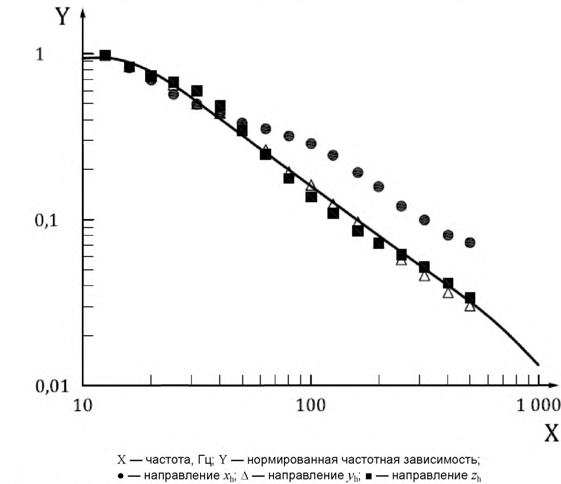
Рисунок F.1 — Сравнение функции частотной коррекции из [2] с частотными зависимостями поглощения мощности системой «кисть — рука» в направлениях x_h , y_h и z_h
