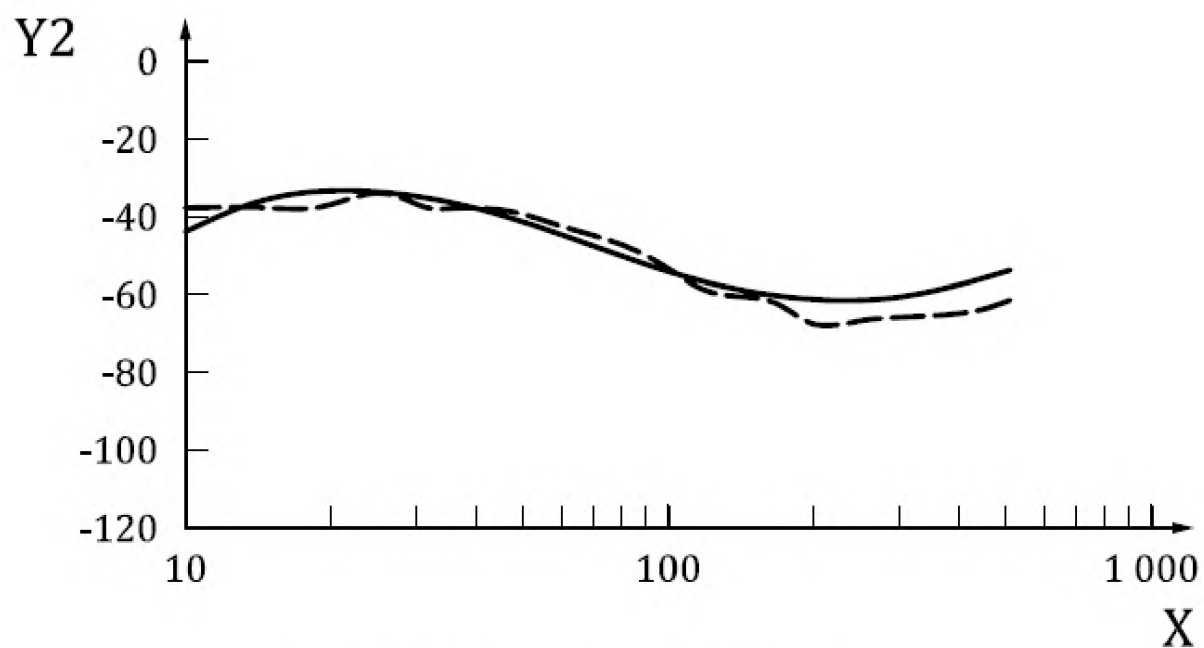
Рисунок В.2 — Сравнение результатов моделирования (сплошная линия) и опорных значений (пунктирная линия) эффективной массы системы «кисть — рука» в направлении x_h
