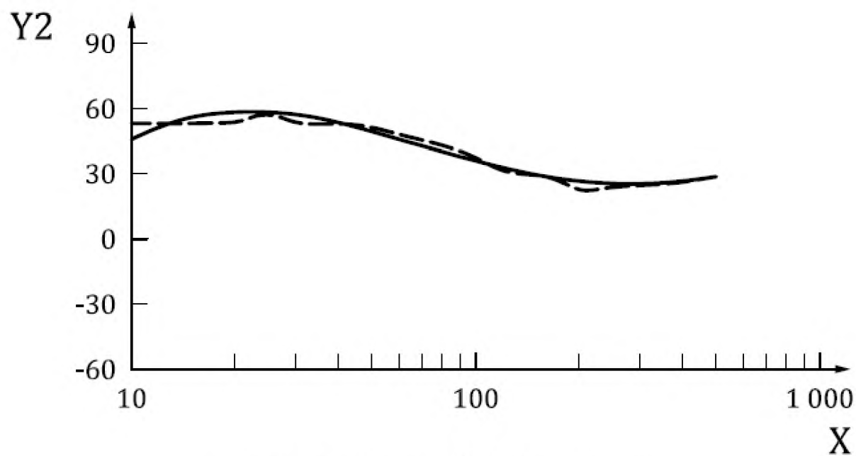
Рисунок С.2 — Сравнение результатов моделирования (сплошная линия) и опорных значений (пунктирная линия) механического импеданса системы «кисть — рука» в направлении x_h
