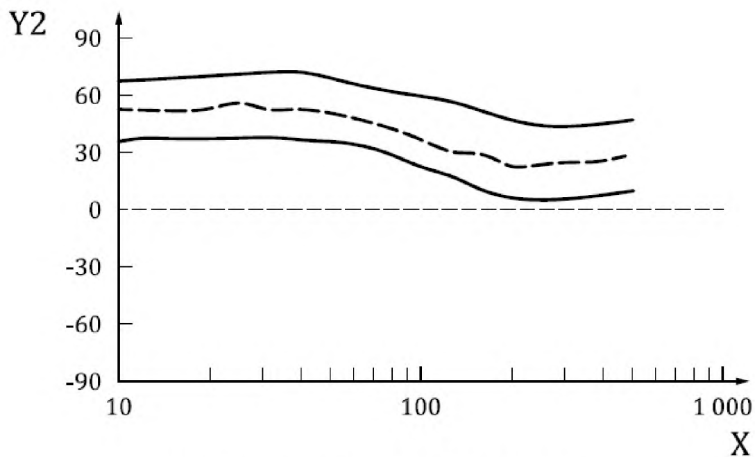
Рисунок 1 — Значения входного механического импеданса для системы «кисть — рука» в направлении x_h
