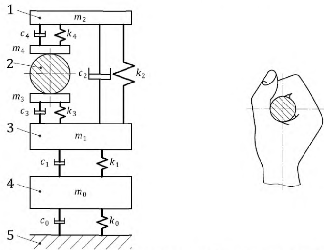
1 — пальцы; 2 — рукоятка; 3 — ладонь, запястье и предплечье; 4 — верхняя часть руки; 5 — верхняя часть тела
