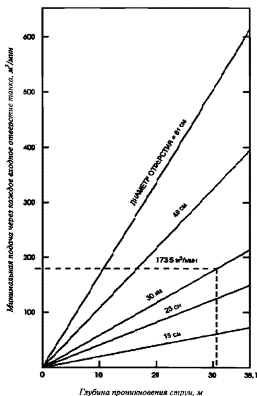
Рис. 4.1.2.1 Зависимость значения минимальной подачи от глубины проникновения струи воздуха в танк
