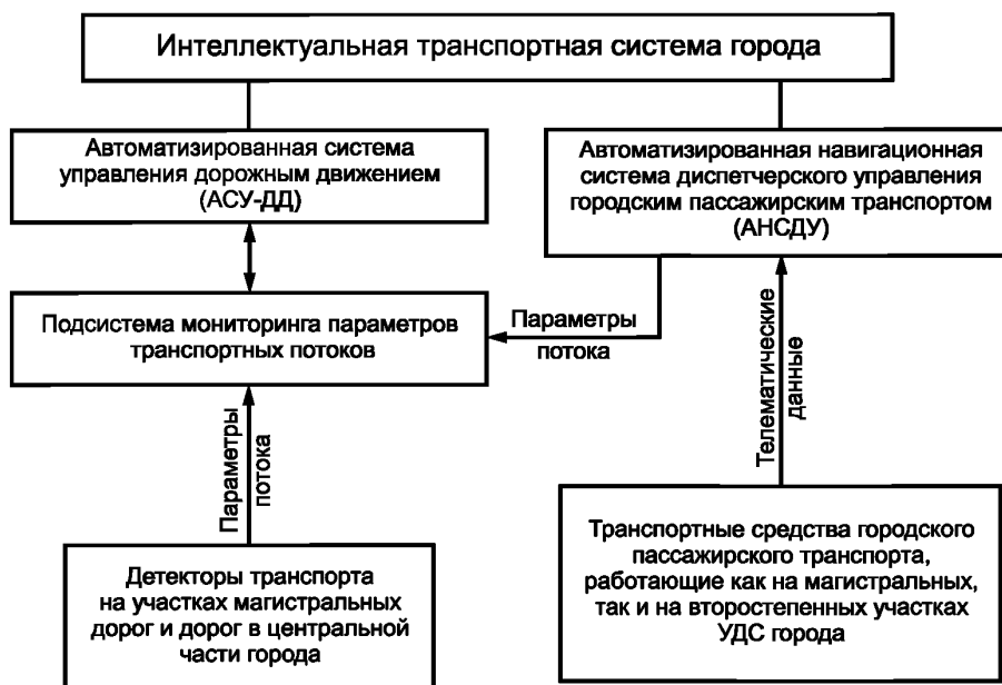
Рисунок 1 — Архитектура подсистемы мониторинга параметров транспортных потоков и ее взаимодействие с другими подсистемами ИТС города
