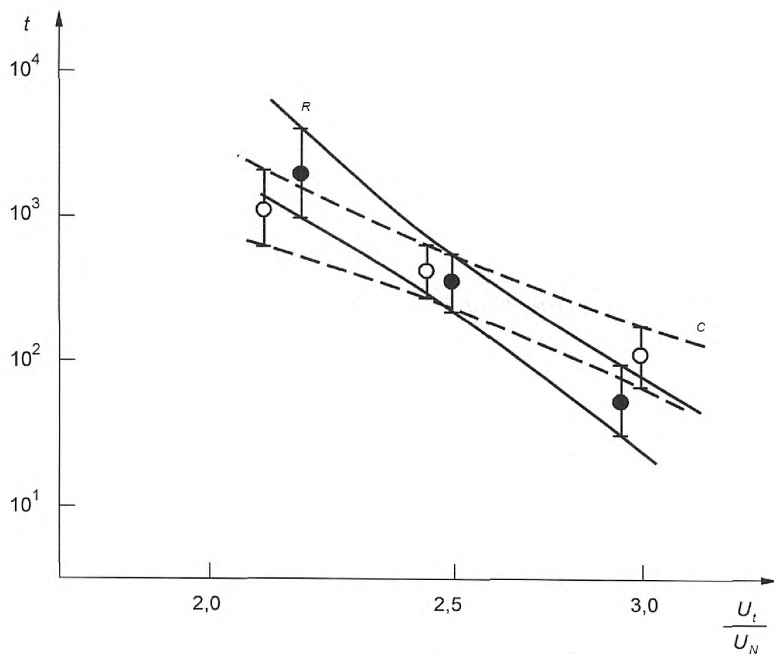
R — данные старения эталонной системы изоляции ( R ) с демонстрацией 90 % доверительного интервала; C — данные старения испытываемой системы изоляции ( C ) с демонстрацией 90 % доверительного интервала; t — время в часах; U_t/U_N — отношение испытательного напряжения к номинальному
