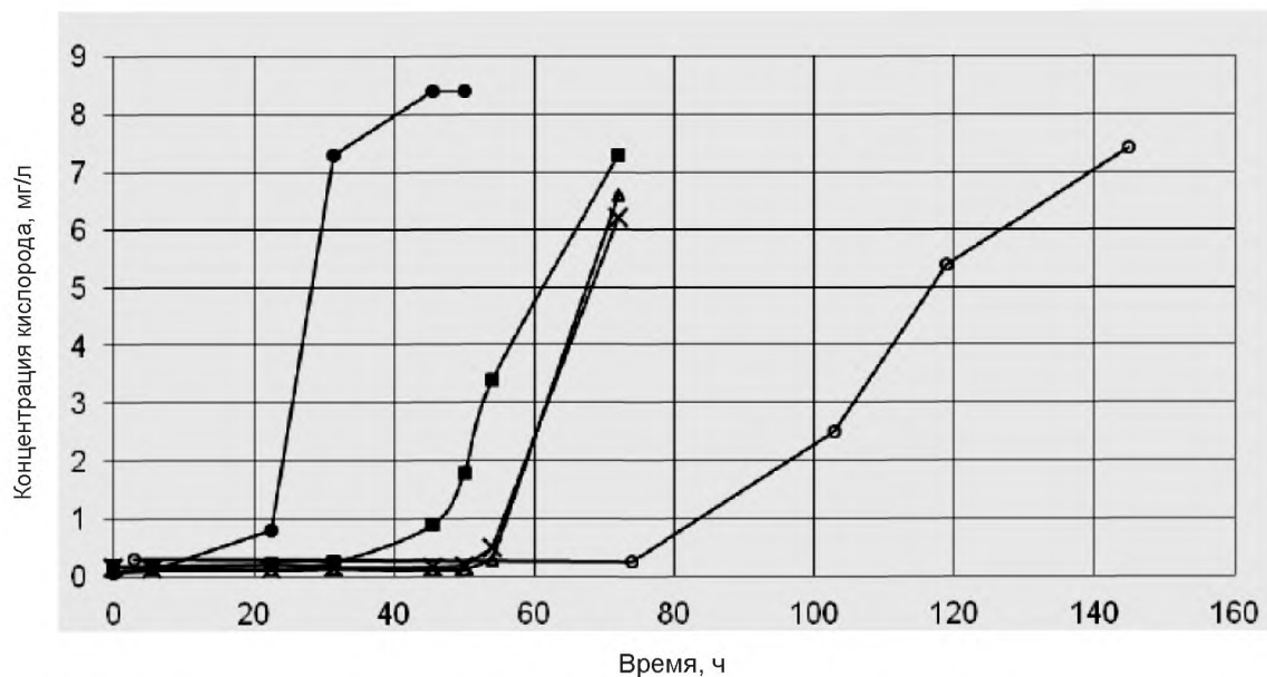
Рисунок 1 — Зависимость от времени концентрации растворенного кислорода при содержании сульфита натрия 2, 4 и 6 г/л в деминерализованной воде для емкостей различного объема и площади поверхности воды
