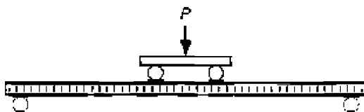
Рисунок 1 — Испытываемый образец и приспособление для проведения испытания
