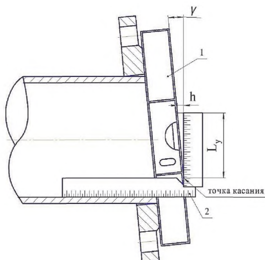
Рисунок 1 — Схема измерений неперпендикулярности
