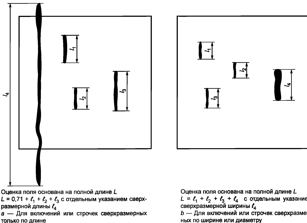
Рисунок В.2 — Оценка поля со сверхразмерными включениями или строчками
