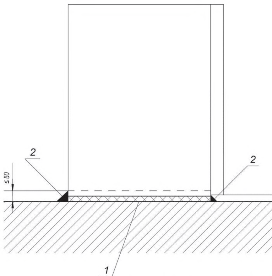
1 — минеральная вата или аналогичный материал; 2 — круговой отлив из огнеупорного раствора
