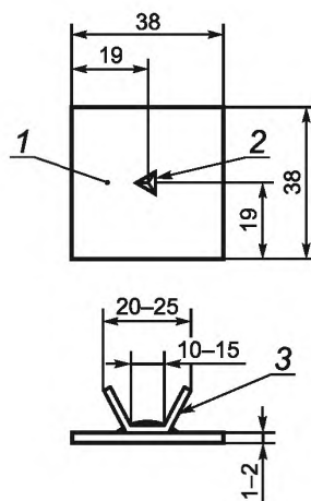
1 — пластинка; 2 — трехгранный керн (глубина керна 0,5—0,7 мм, угол наклона между плоской гранью и осью керна 60^\circ ); 3 — медные анкера с припоем
