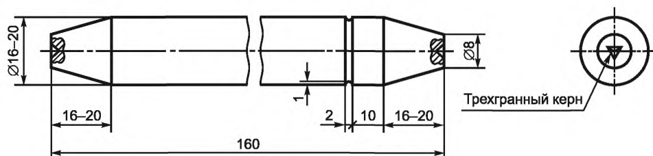
Рисунок 1 — Эталон длины
