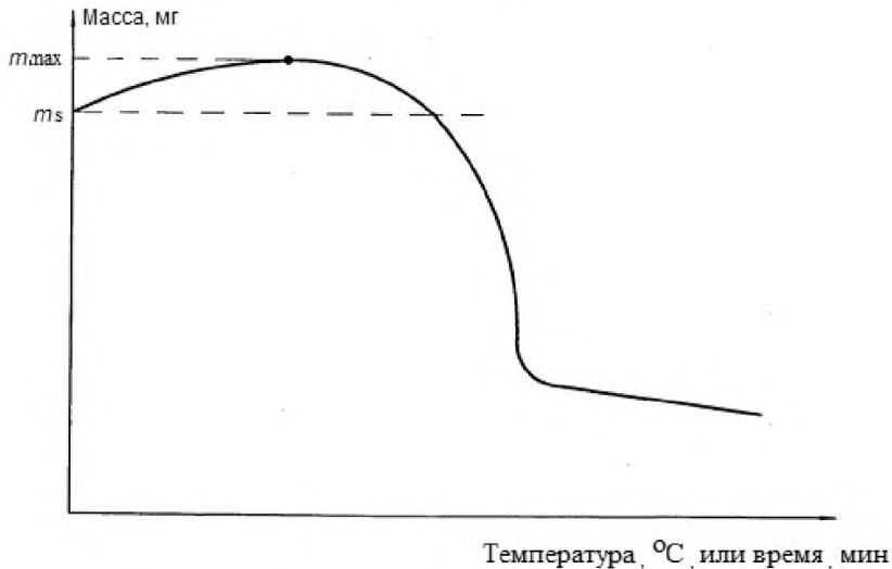
Рисунок 1 — Пример ТГ кривой, показывающей увеличение массы образца
