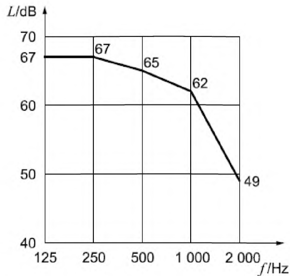
Рисунок 2 — Оценочная кривая для ударного шума (октавные полосы)
