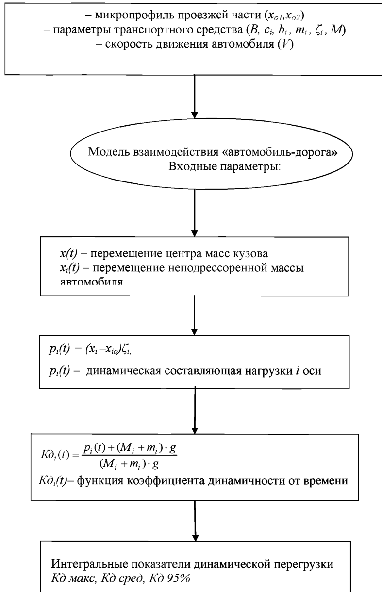
Рисунок 6.3 Расчет коэффициента динамичности на участке автомобильной дороги
