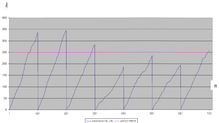
Рисунок 5.5 Типовой график ровности с накоплением, полученный передвижной дорожной диагностической лаборатории (по вертикали – k - количество сотых мм)
