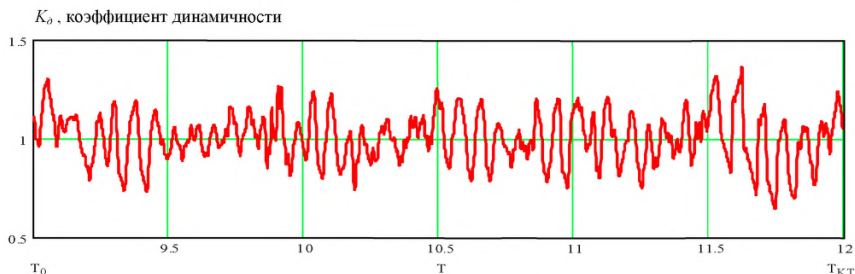
Рисунок 6.1 Амплитудно-временная характеристика коэффициента динамичности
