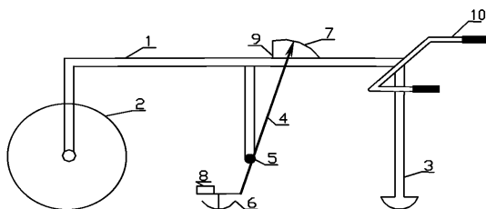
Рисунок 5.6 - Общий вид измерительного устройства «Мерлин»: 1 – рама; 2 – колесо; 3 – стойка с криволинейным основанием; 4 – рычаг; 5 – ось; 6 – зонд; 7 – указатель; 8 – груз; 9 – крепление листа; 10 – ручки
