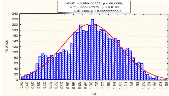
Рисунок 6.2 Гистограмма распределения коэффициента динамичности на участке Азов-Староминская км 45 при проезде автомобиля ВА3-21213 со скоростью 100 км/ч
