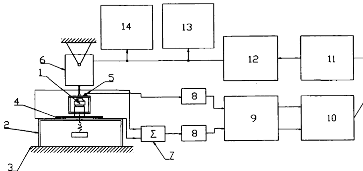
Рисунок 6.11 Экспериментальный стенд для динамических испытаний:
