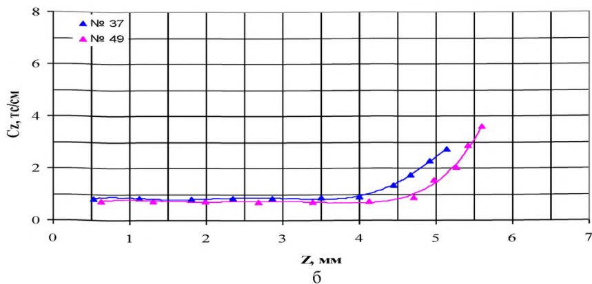
Статическая жесткость для одного образца гидропоры в осевом направлении Z
