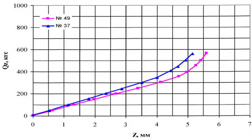
Статическая жесткость для одного образца гидропоры в осевом направлении Z
