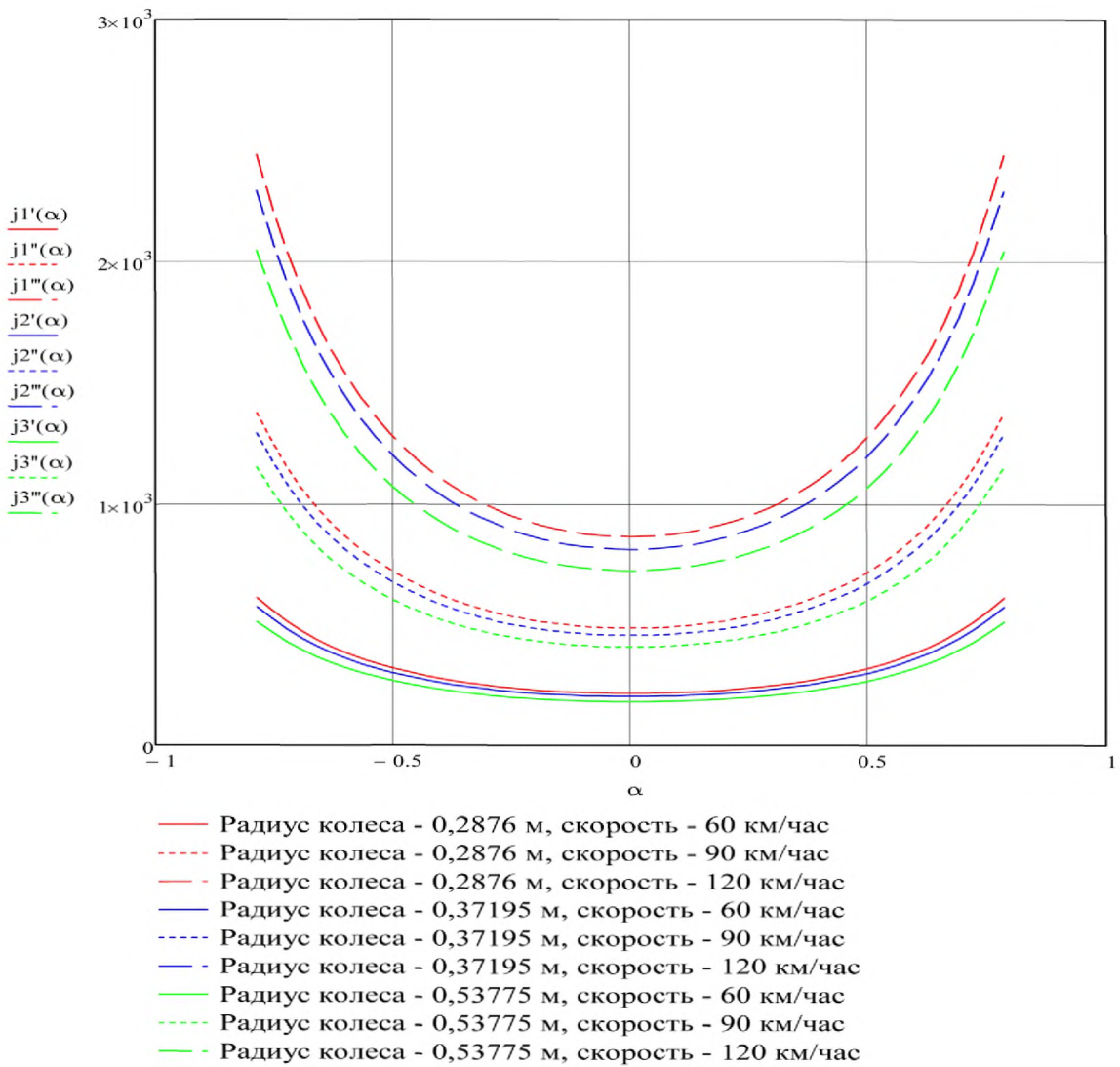
Рисунок П.2 Результаты работы программного комплекса имитационного моделирования процесса динамического взаимодействия колеса транспортного средства и дорожного покрытия с единичными и накопленными неровностями в среде МАТЛАБ
