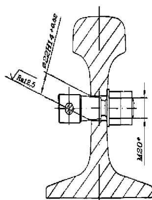
Крепление перемычки к рельсу
