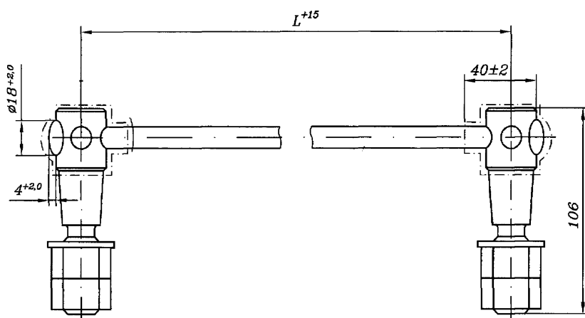
Рисунок 1.8.1 Внешний вид соединителя
