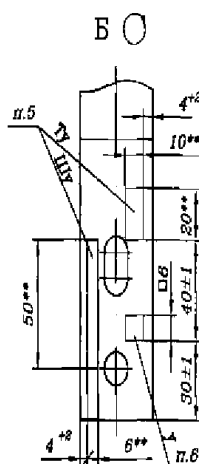
Крепление перемычки к рельсу
