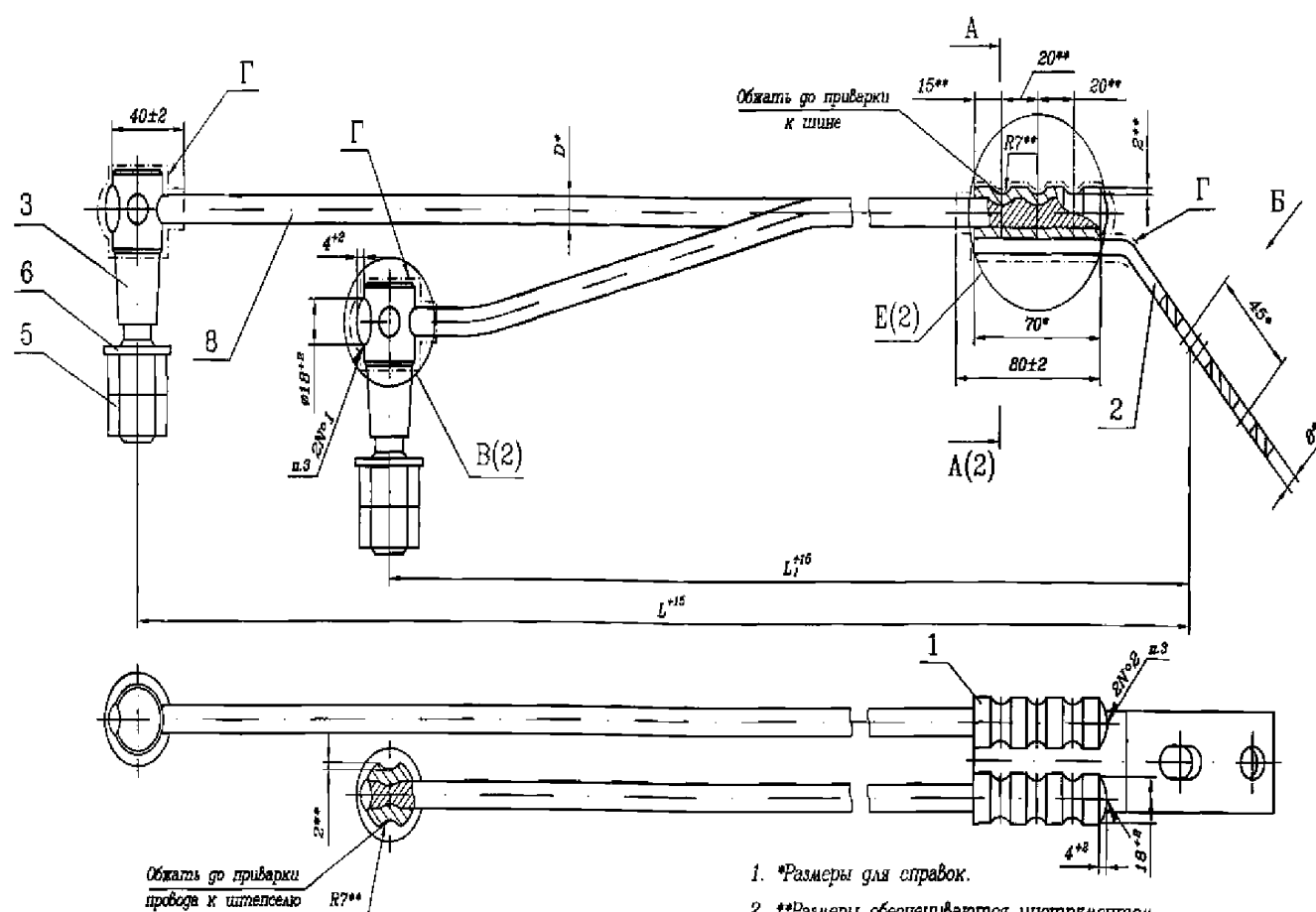
Крепление перемычки к рельсу
