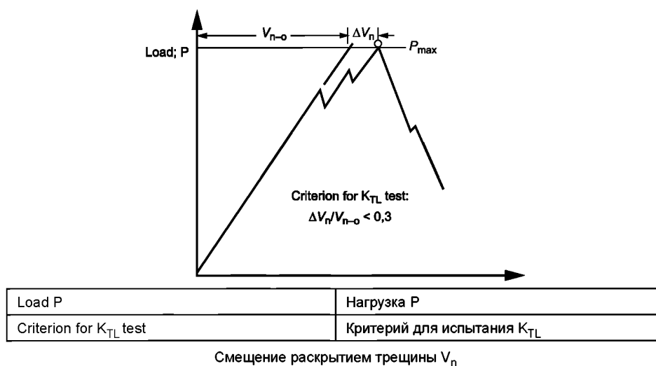
Рисунок 3 — Типовой график зависимости нагрузки от смещения раскрытием трещины
