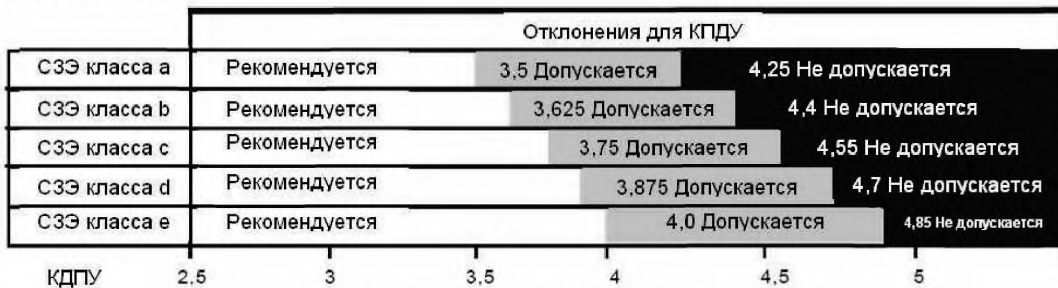
Рисунок 15 — Рекомендации по выбору коэффициента длины пути утечки
