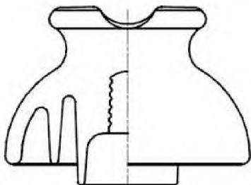
Рисунок 6а — Цельный штыревой изолятор
