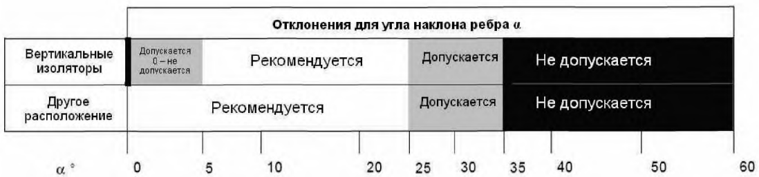
Рисунок 14б — Рекомендации по выбору угла наклона ребра
