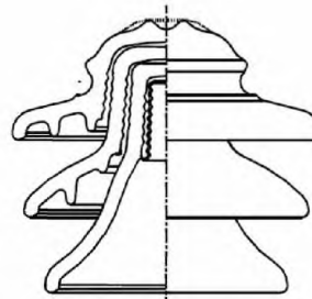
Рисунок 6б — Многоэлементный штыревой изолятор
