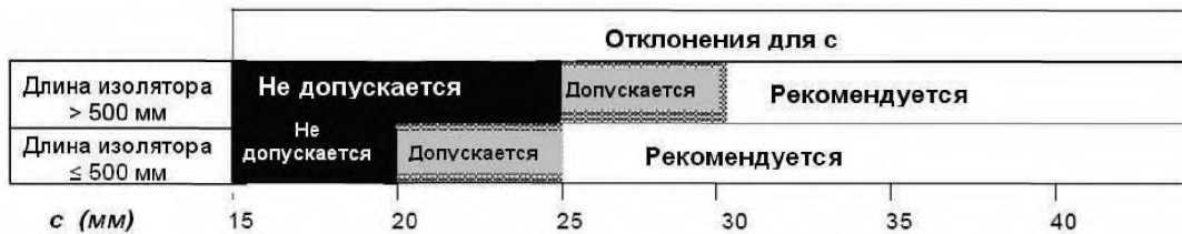
Рисунок 11 — Рекомендации по выбору межреберного расстояния
