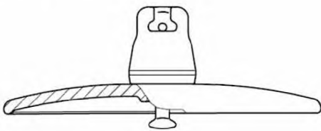
Рисунок 3а — Аэродинамические тарельчатые изоляторы
