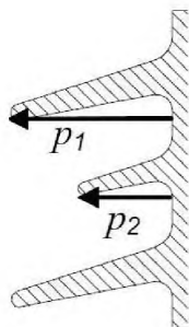
Рисунок 7 — Переменный профиль ребер
