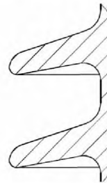
Рисунок 2б — Стандартный профиль ребра — длинностержневые, опорные и полые изоляторы
