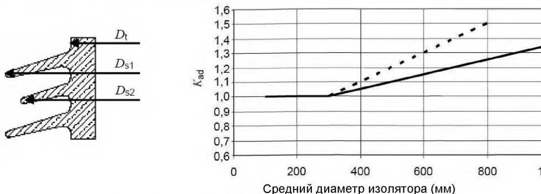
Рисунок 16 — K_{ad} в зависимости от диаметра изолятора
