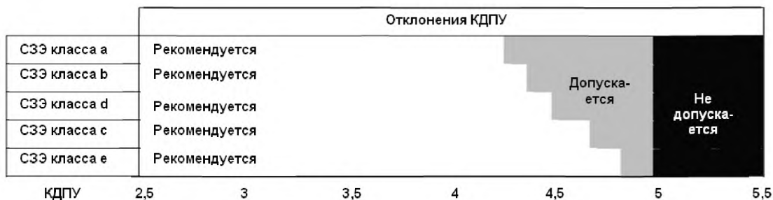
Рисунок 16 — Рекомендации по выбору коэффициента длины пути утечки
