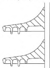
Рисунок 5 — Типичный профиль с глубокими канавками под ребром
