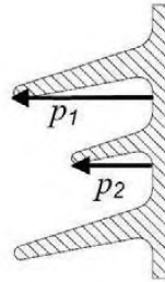
Рисунок 7 — Переменный профиль ребер
