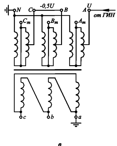
Рисунок DA.2.6 — Пофазное испытание трехобмоточного автотрансформатора
