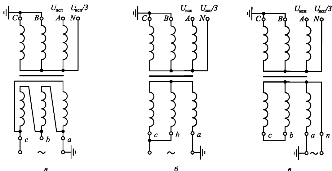
Рисунок ДА.3.1 — Пофазное испытание трехфазного трансформатора
