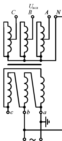
Рисунок ДА.3.6 — Испытание фазы В с подпором от обмотки испытываемого трансформатора
