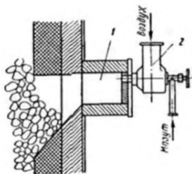
1 — форкамера; 2 — мазутная форсунка
