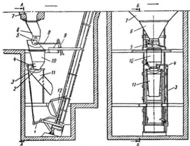
1, 3, 4 и 8 — рычаги; 2 — затвор; 5 — затвор течки; 6 и 11 — течки; 7 — бункер; 9 — рычаг с вилкой; 10 — дозирующий бункер; 12 — бункер
