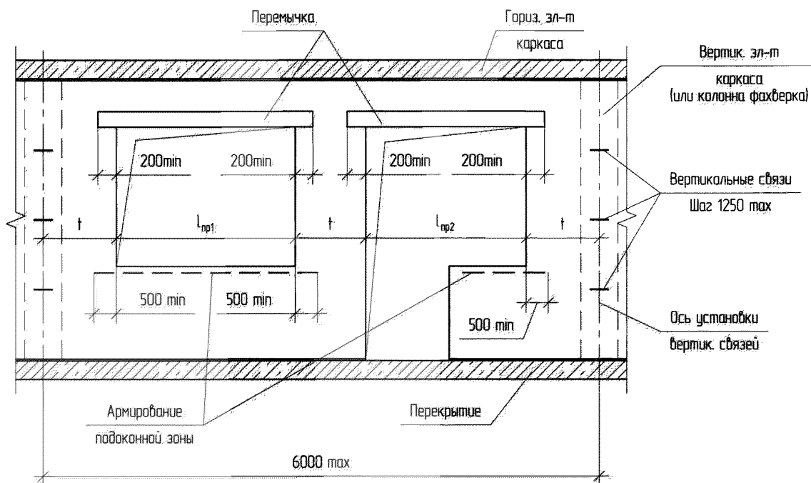
Рис. 4.8. Схема устройства проемов на примере наружной стены
