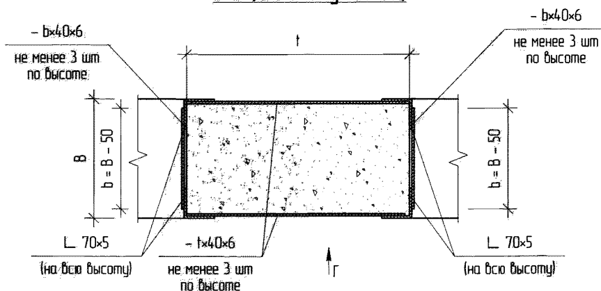
5-5 (см. схему XII-06.)
