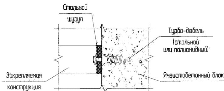
б) Винтовой турбо-дюбель для газобетона
