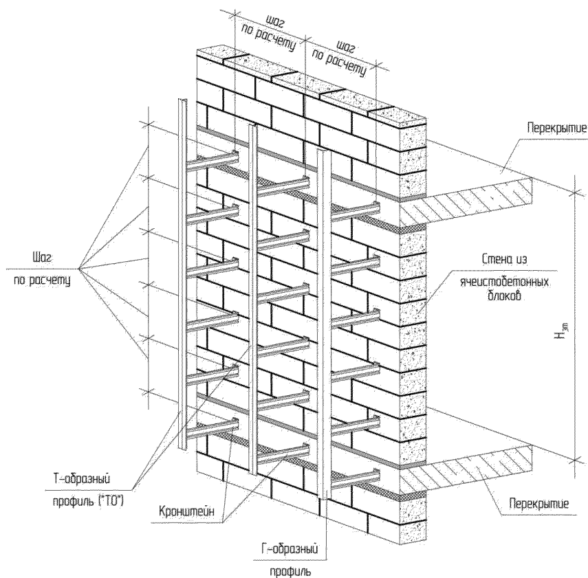
а) При помощи кронштейнов и вертикальных направляющих
