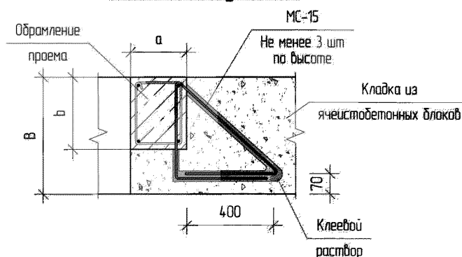
4-4 (см. схему XII-Об.)
