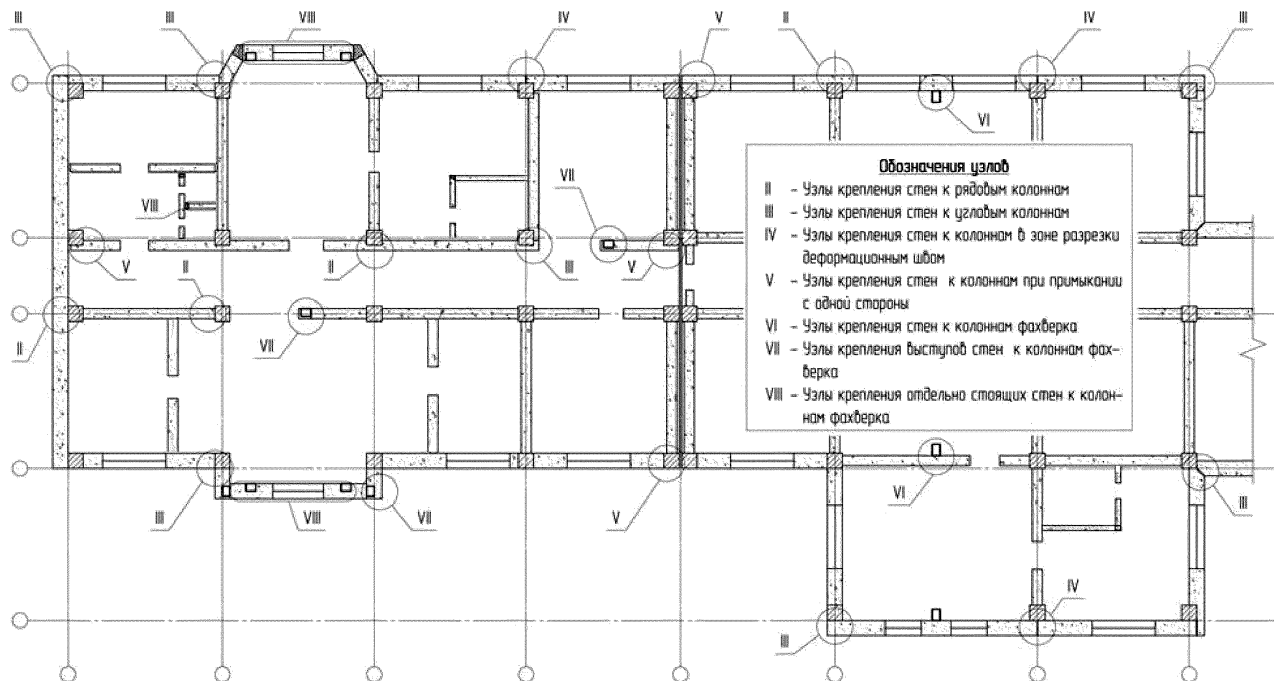
Рис. 4.7. Маркировочная схема узлов связей наружных стен с несущими вертикальными конструкциями
