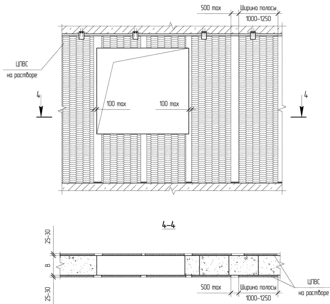
Рис. 3.10. Схема вертикального армирования стен цельнометаллическими просечно-вытяжными сетками
