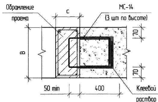
3-3 (см. схему X-0б.)
