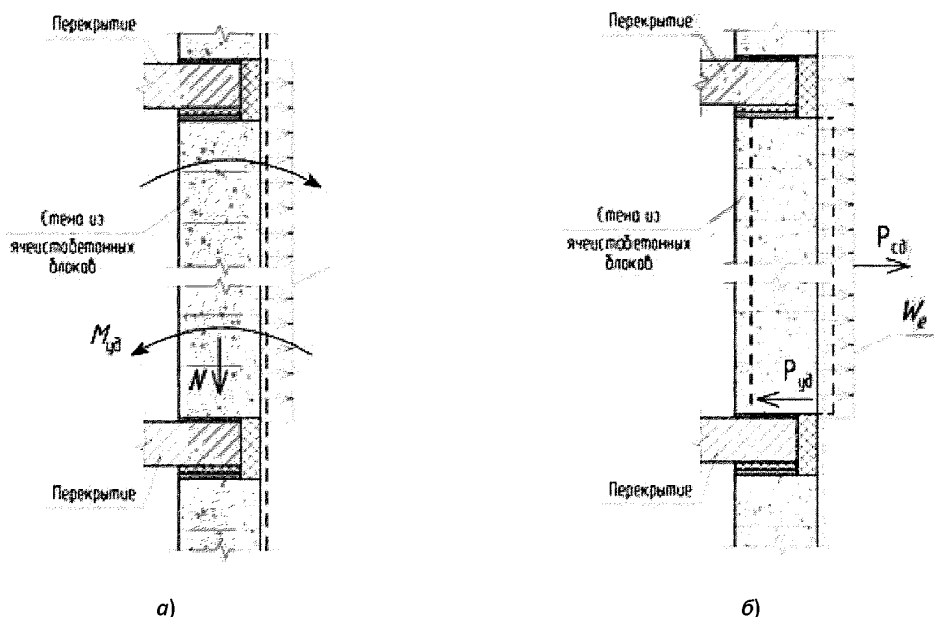
Рис. 3.14. Расчетные схемы поэтажно опертой стены
