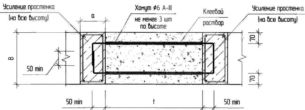
5-5 (см. схему XII-0б.)
