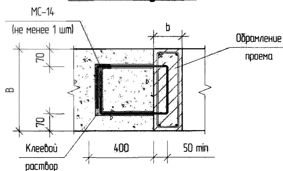
3-3 (см. схему X-0б.)
