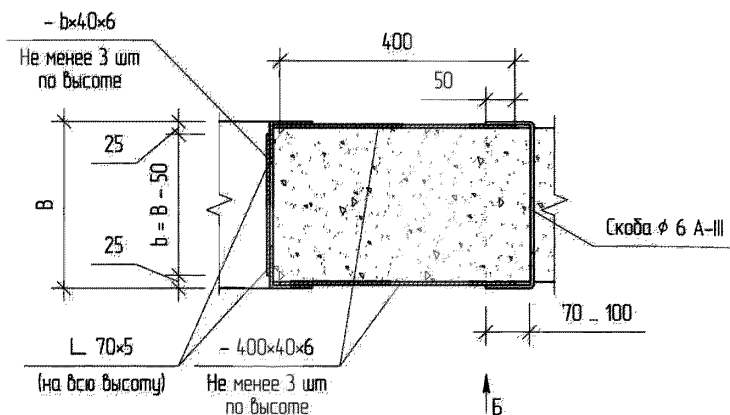
4-4 (см. схему XII-0б.)
