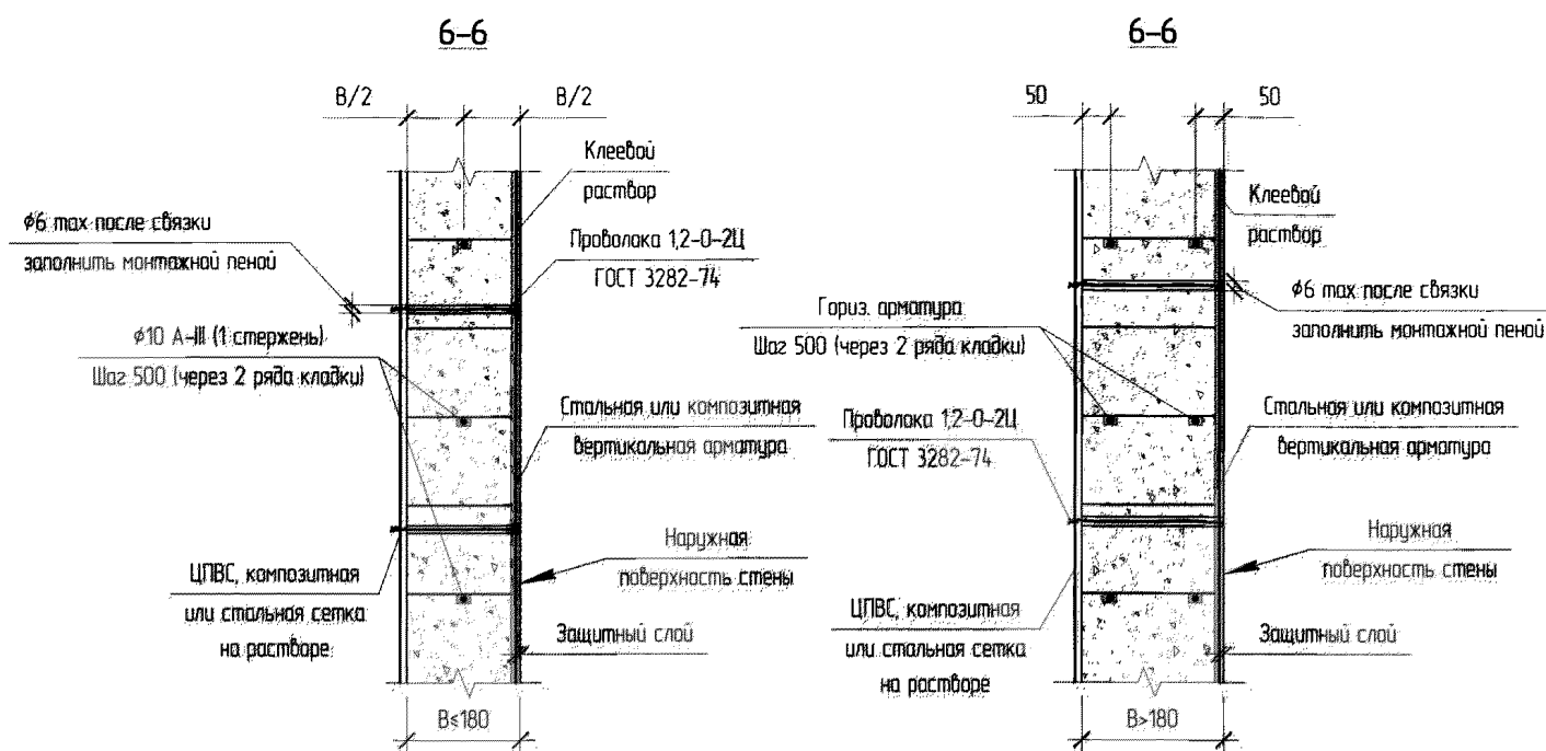
Рис. 3.12. Вертикальное армирование стен по схеме: «отдельные стальные стержни с наружной стороны – ЦПВС или сетки с внутренней стороны»
