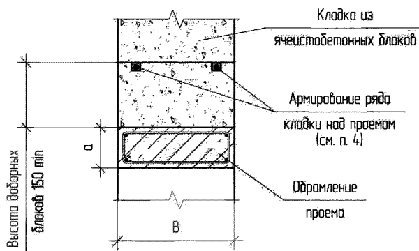
2-2 (см. схему X-Об.)
