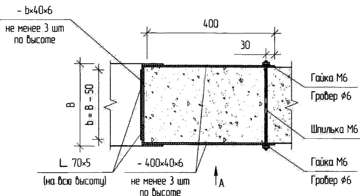
4-4 (см. схему XII-03.)
