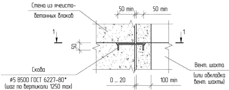
А (см. схему XVI-0. 1/1)
