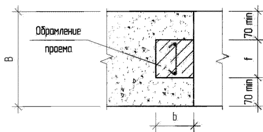
4-4 (см. схему XII-0б.)
