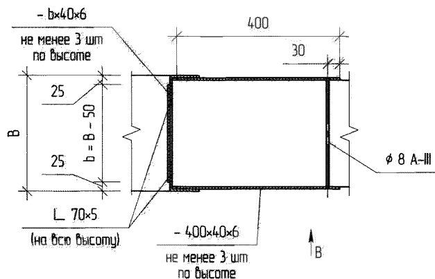
4-4 (см. схему XII-05.)
