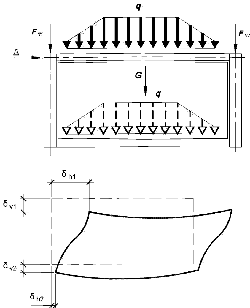
Рис. 3.13. Схемы для определения нагрузок
