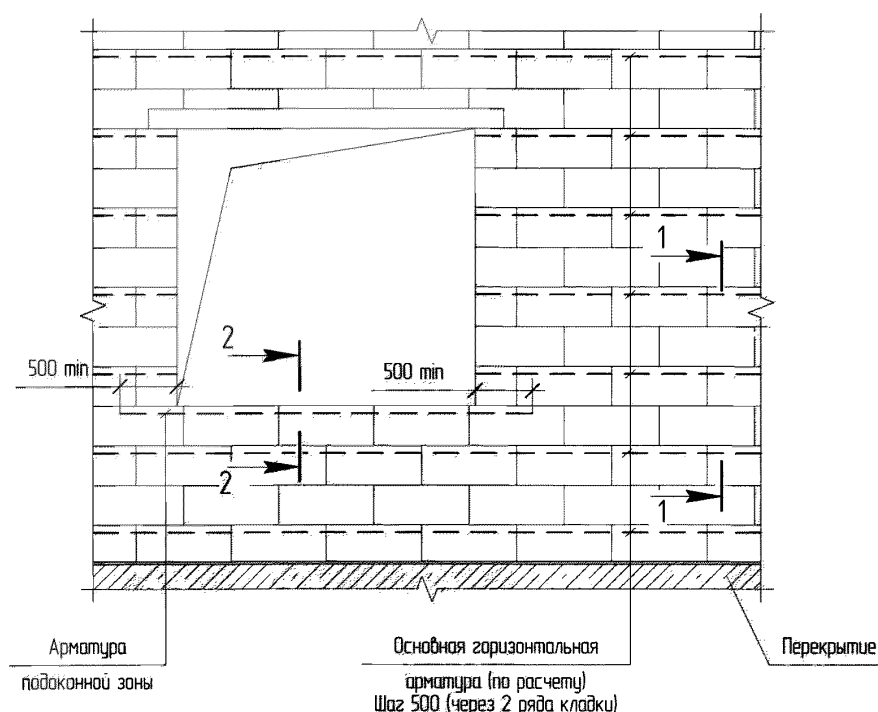
Рис. 3.4. Общая схема горизонтального армирования стен
