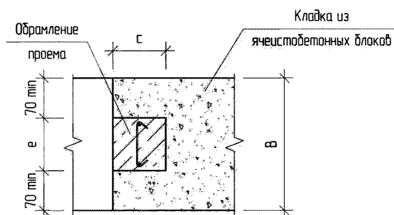
4-4 (см. схему XII-0б.)
