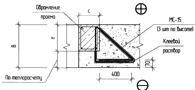
3-3 (см. схему X-Об.)
