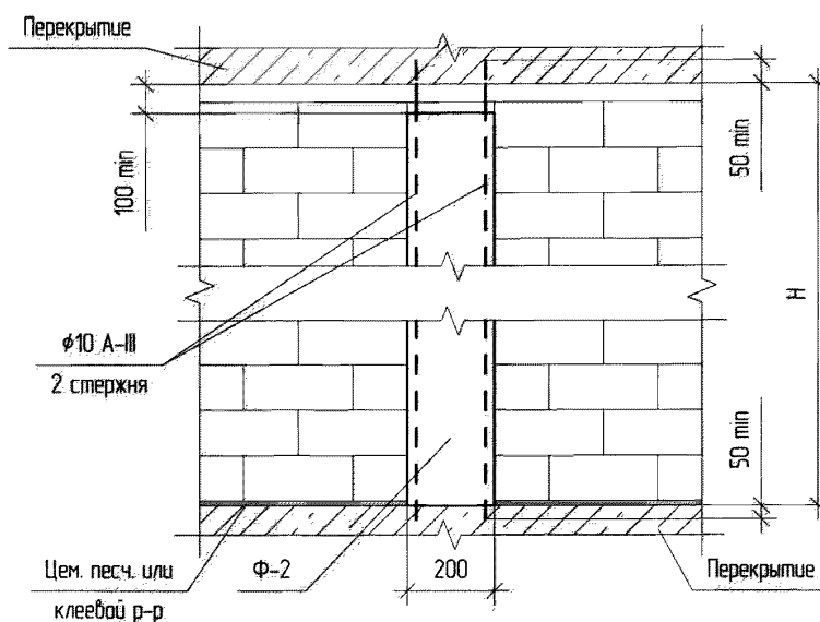
Вид А (заделка горизонтального шва не показана)
