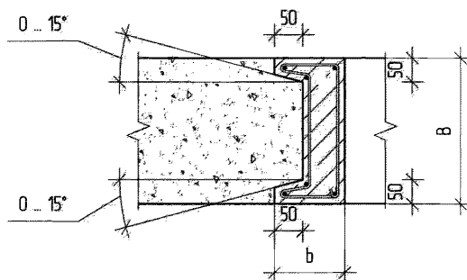
3-3 (см. схему X-0б.)
