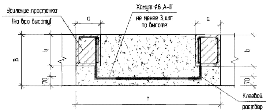
5-5 (см. схему XII-0б.)
