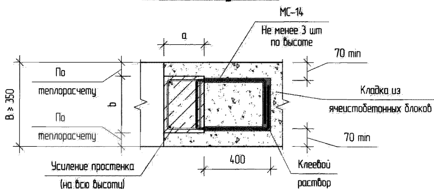
4-4 (см. схему XII-Об.)
