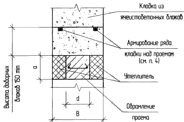
2-2 (см. схему X-0б.)
