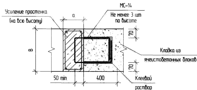
4-4 (см. схему XII-Об.)
