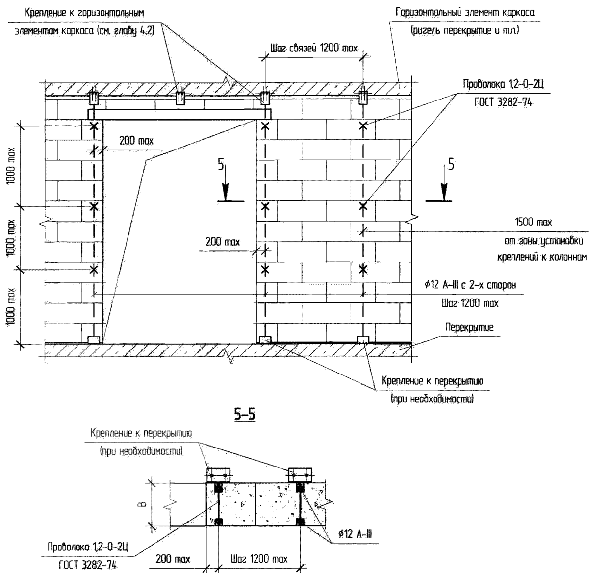
Рис. 3.11. Схема вертикального армирования стен отдельными арматурными стержнями
