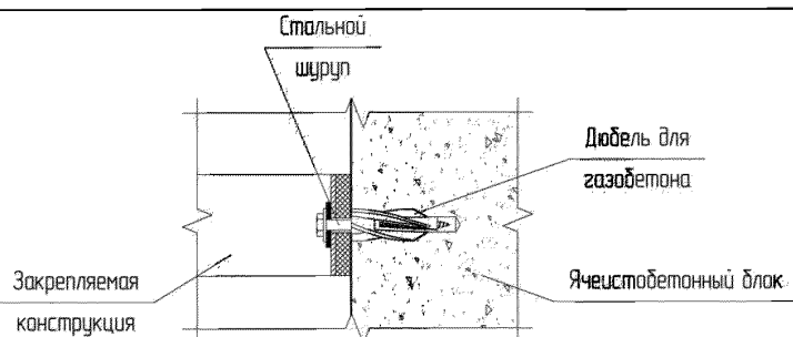
а) Винтовой дюбель для газобетона
