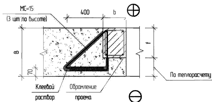
3-3 (см. схему X-Об.)
