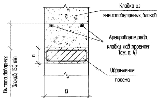
1-1 (см. схему X-Об.)
