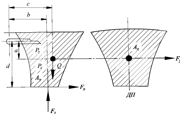
Вид сбоку
