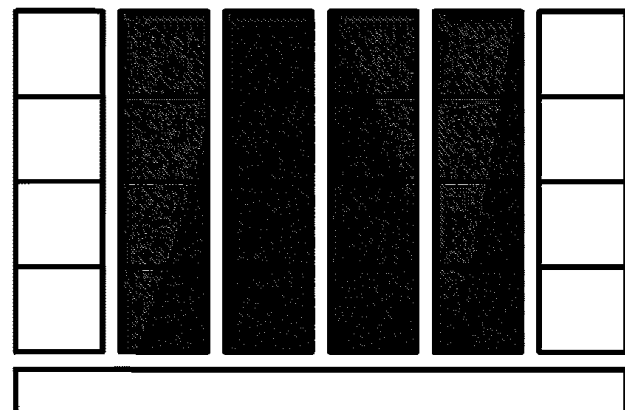
Рис 7.10.6.12 Частичная нагрузка на крышку контейнерного трюма
