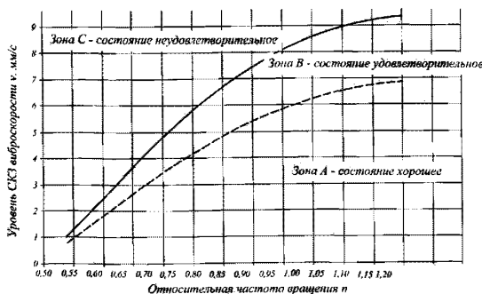
Рис. 9.9.3 Нормы вибрации винторулевых колонок
