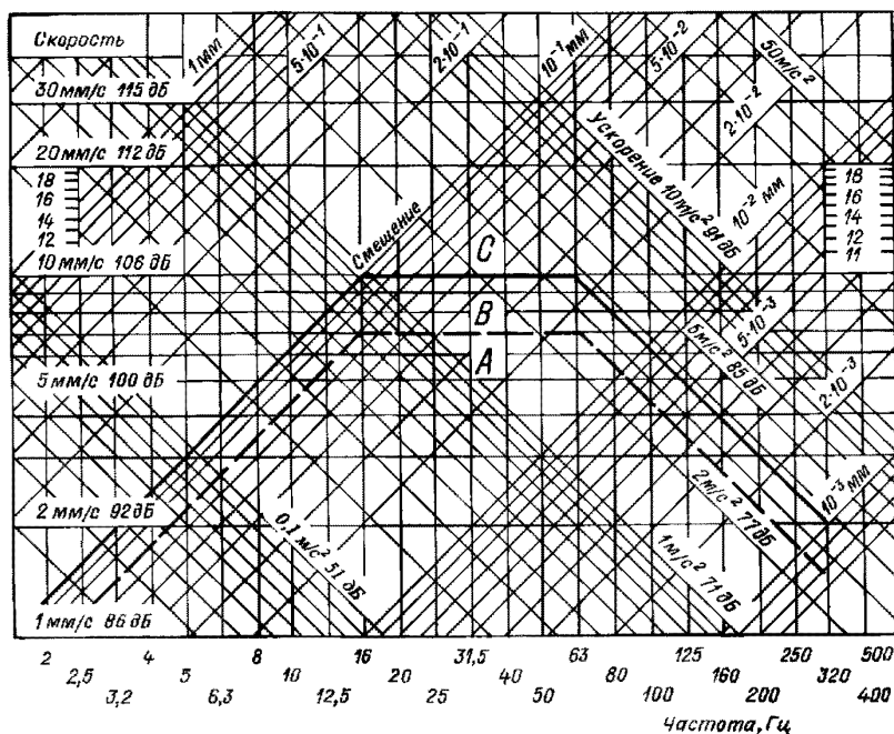
Рис. 9.7.1 Нормы вибрации котлов, вспомогательных механизмов и оборудования:
