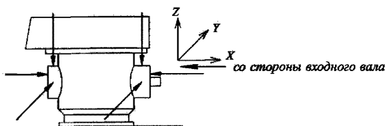
Рис. 9.9.2 Точки измерения вибрации винторулевых колонок
