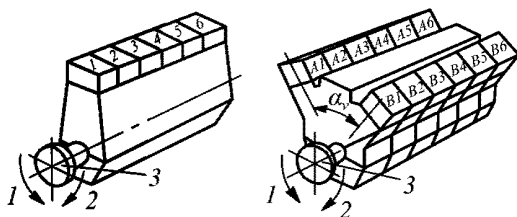
Рис. 2.4.3-1 Направления вращения коленчатого вала: 1 — против часовой стрелки; 2 — по часовой стрелки; 3 — фланец отбора мощности
