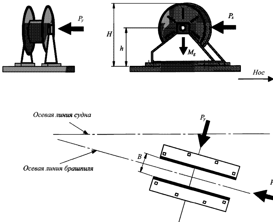
Рис. 6.3.5.3 Направление сил
