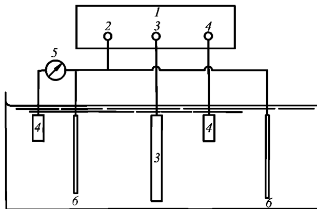
Рис. 2.5.6.1-1 Потенциостатически контролируемая катодная защитная цепь:
