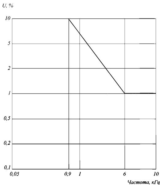
Рис. 5.1.43.3 Кривая испытательного напряжения при проверке оборудования на устойчивость к низкочастотным кондуктивным помехам
