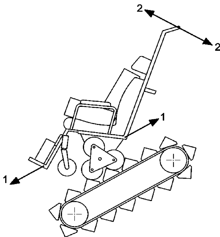
Рисунок F.2 — Устройство для преодоления лестниц, стабилизируемое вручную, на эскалаторной испытательной машине
