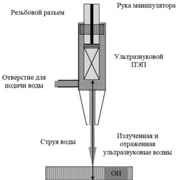
Рисунок 1 — Метод А. Автоматизированный ультразвуковой эхо-импульсный метод
