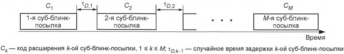
Рисунок 4 — Основной принцип передачи пакетов данных с использованием кодовых пар с несколькими кодами расширения
