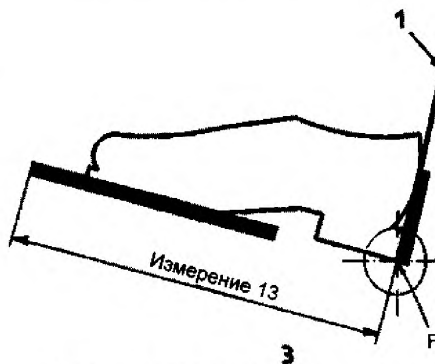
б) Длина опоры стопы с задником-держателем
