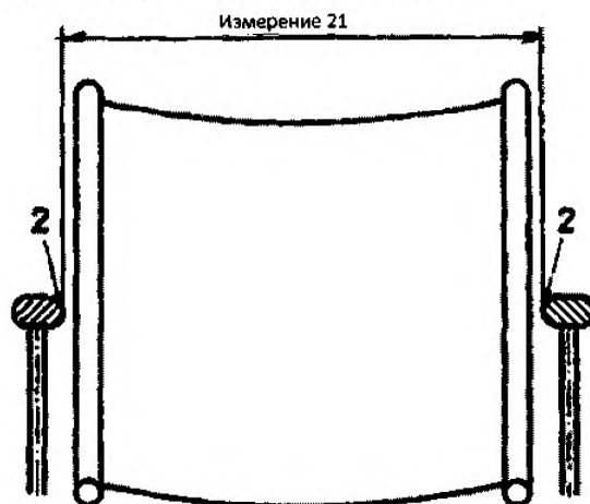
Рисунок 30 — Расстояние между подлокотниками
