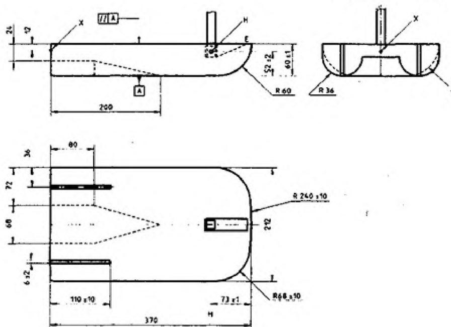
Рисунок А.4 — Узел сиденья ЭНУР
