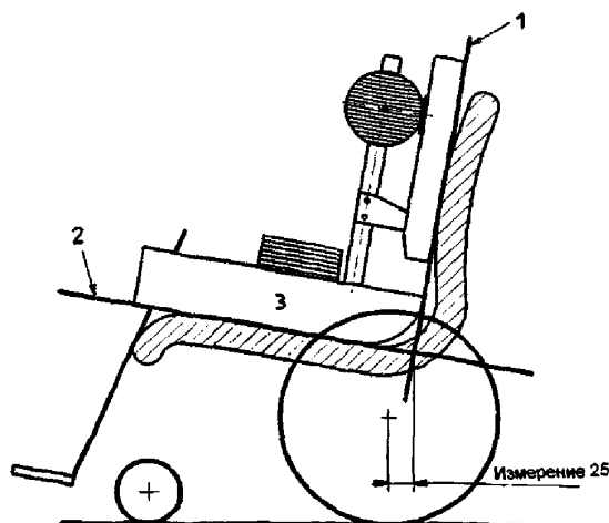
а) Горизонтальное положение оси ведущего колеса
