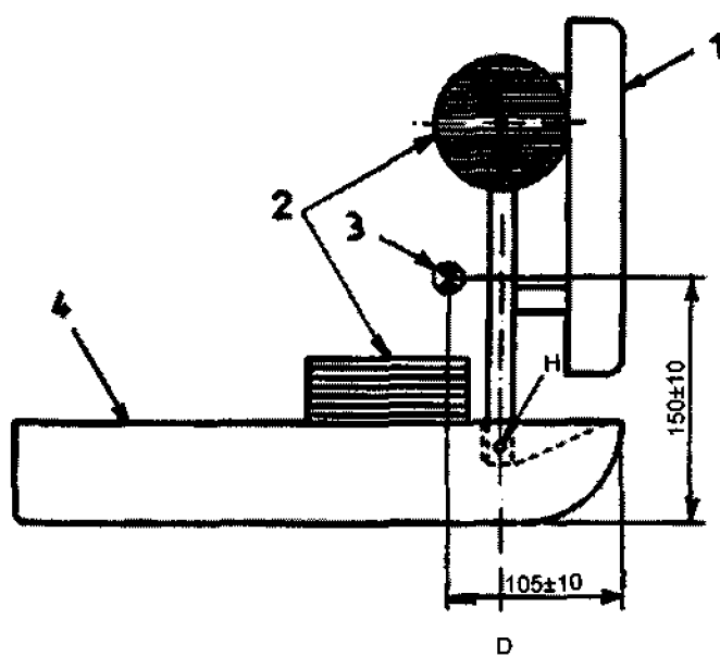
Рисунок А.6 — Положение центра тяжести ЭНУР
