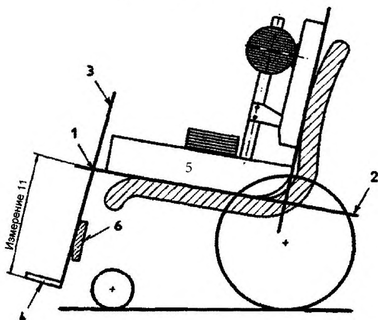
Рисунок 20 — Длина подножки
