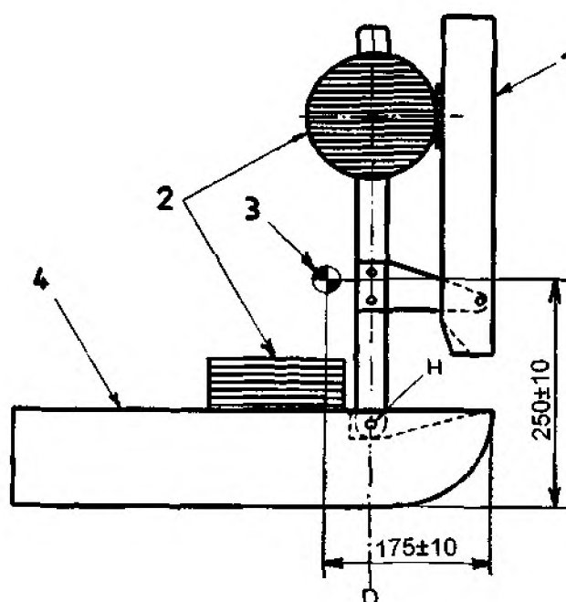
Рисунок А.3 — ЭНУВ — Положение центра тяжести
