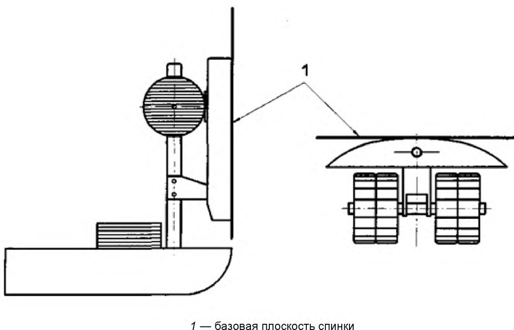
Рисунок 2 — Базовая плоскость спинки
