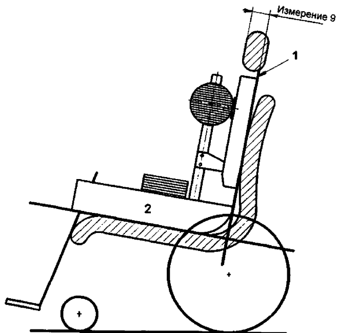
1 — базовая плоскость спинки; 2 — ЭНУ
