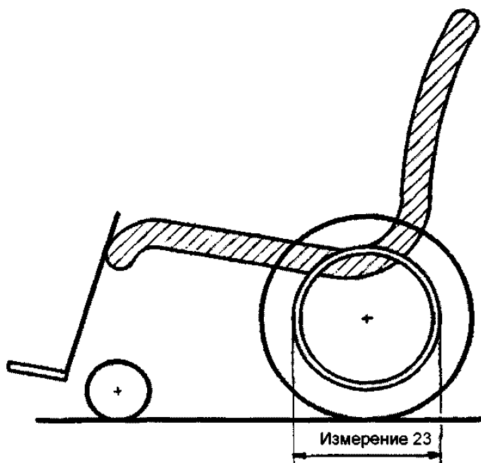
Рисунок 32 — Диаметр обода ручного привода
