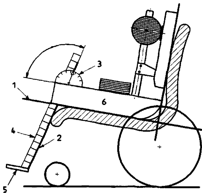
б) Измерение угла наклона подножки
