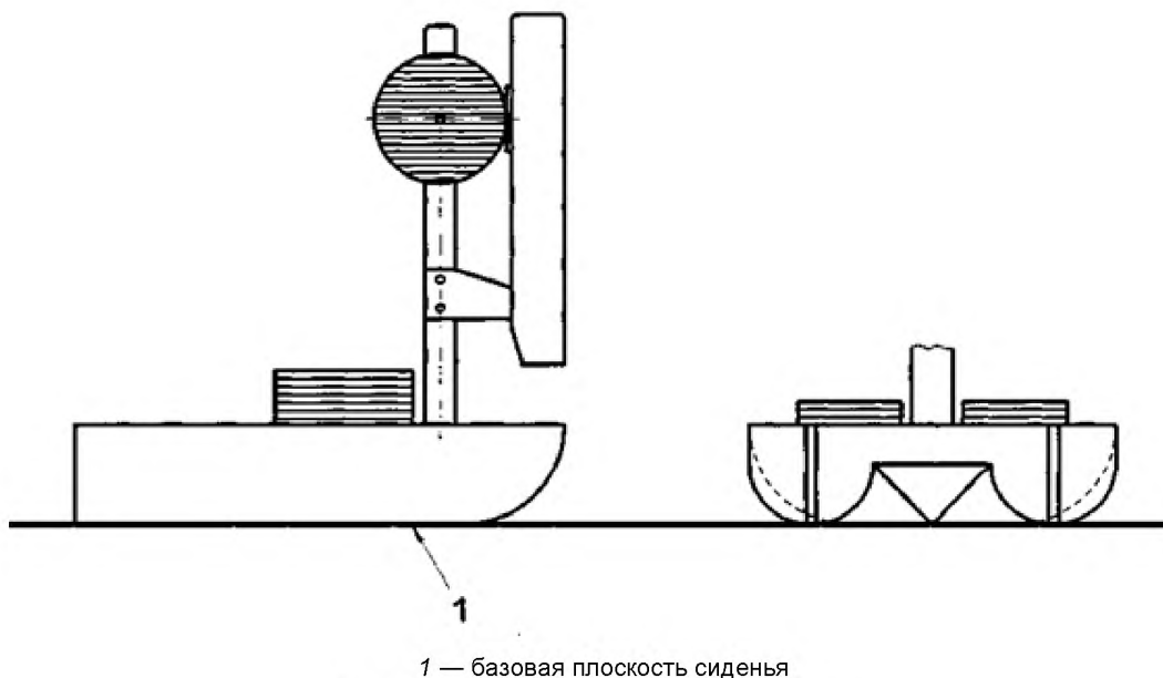
Рисунок 1 — Базовая плоскость сиденья
