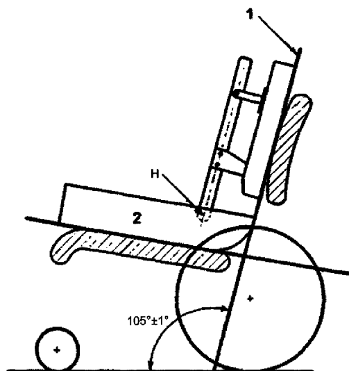
1 — базовая плоскость спинки; 2 — ЭНУ
