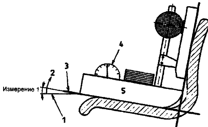
1 — горизонталь; 2 — положительное направление; 3 — базовая плоскость сиденья;
