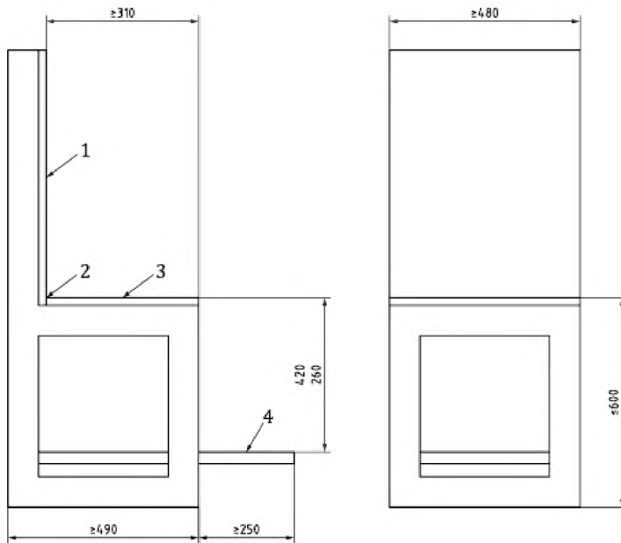
Рисунок 1 — Испытательное приспособление
