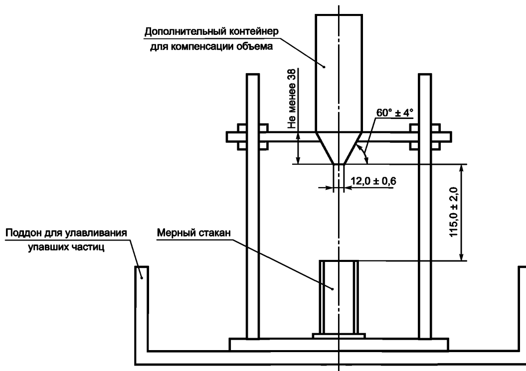
Рисунок 2 — Схема расположения воронки со стойкой и мерного стакана
