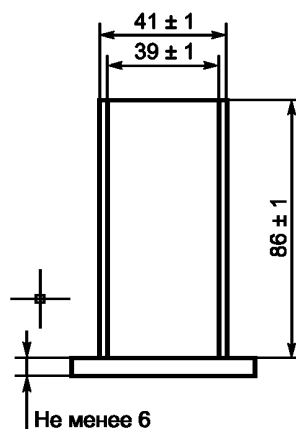
Рисунок 1 — Мерный стакан емкостью 100 мл
