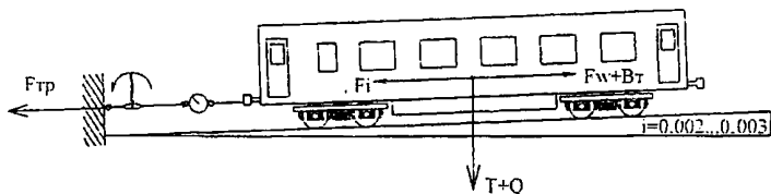
Рис. А.13. Схема приложения сил к объекту испытаний
