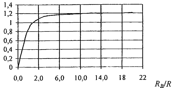
Рисунок А.9 Графики для определения коэффициента учета внешних динамических нагрузок на якорные подшипники K_{ЭВ}
