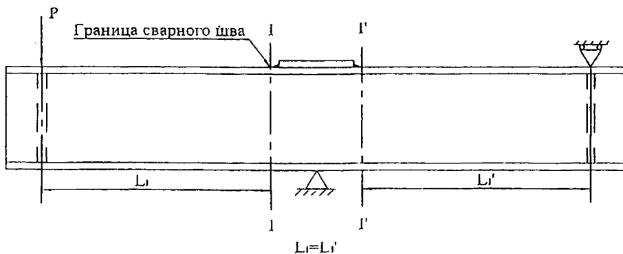
Рисунок А.6 Схема нагружения типового сварного образца (точка приложения пульсирующей нагрузки P может быть изменена в зависимости от конструкции стенда)
