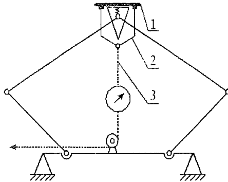
Рис. А.16. Схема для определения аэродинамической характеристики токоприемников:
