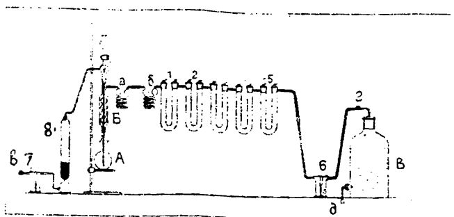
Рис. I. Прибор для прямого определения двуокиси углерода.
