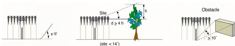
Рисунок А.1 – Место размещения осадкомера при классе 1
