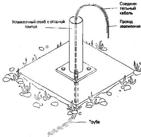
Рисунок Б.2 – Место установки, подготовленное для монтажа осадкомера OTT Pluvio 2 200
