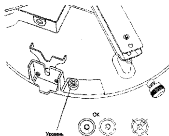
Рисунок Б.3 – Юстировка осадкомера OTT Pluvio 2 200
