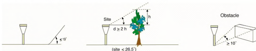
Рисунок А.2 – Место размещения осадкомера при классе 2
