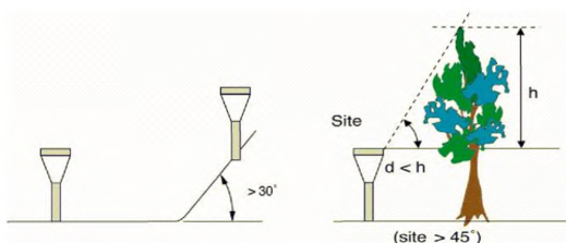
Рисунок А.4 – Место размещения осадкомера при классе 4
