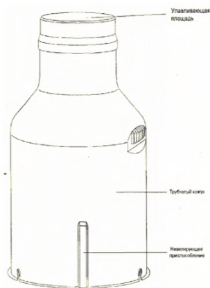
Рисунок 2 – Трубчатый (защитный) кожух осадкомера ОТТ Pluvio 2 200
