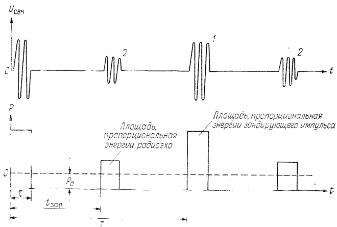
Черт. 1.2. Иллюстрация импульсного метода работы радиолокатора.
