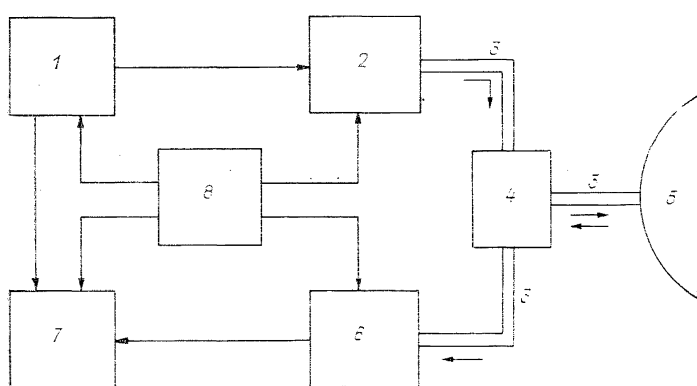
Черт. 1.1. Функциональная схема импульсной радиолокационной станции.
