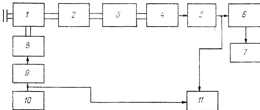
Черт. 7.2. Схема подключения приборов для измерения чувствительности и градуировки системы ступенчатого изоэха МРЛ-2.
