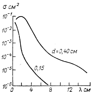
Черт. 1.10. Зависимость эффективной площади рассеяния \sigma водяных сфер разного диаметра от длины волны.
