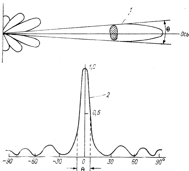
Черт. 1.3. Диаграмма направленности антенны.
