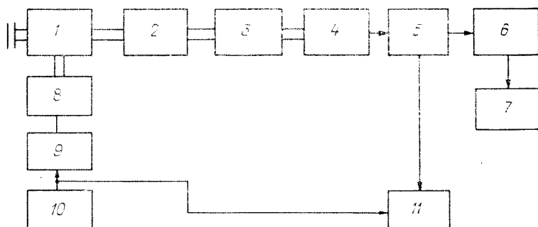
Черт. 7.1. Схема подключения приборов для измерения чувствительности и градуировки системы ступенчатого изоэха МРЛ-1.
