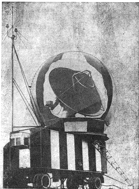
Черт. 6.6. Метеорологический радиолокатор МРЛ-5.
