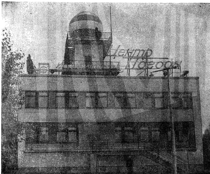
Черт. 6.3. Метеорологический радиолокатор МРЛ-2.
