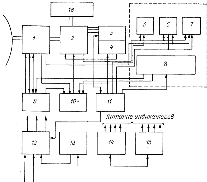
Черт. 6.5. Функциональная схема МРЛ-2.
