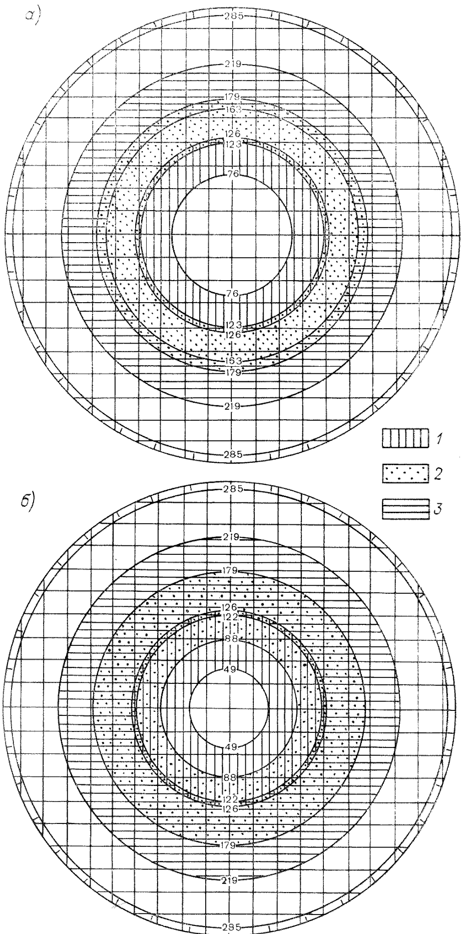
Черт. 2.23. Зоны пересечения диаграммой направлен угла возвышения антенны а) \varepsilon = 0^\circ ; б) \varepsilon = 0,5^\circ ; в) \varepsilon = 1^\circ ; г) \varepsilon = 1,5^\circ . 1) H_0 < C = 1 км;
