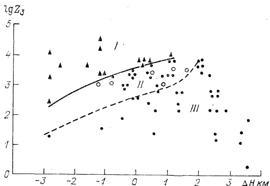
Черт. 5.10. График индикации шкалистых усиления ветра по данным измерений МРЛ.
