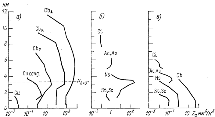
Черт. 2.16. Вертикальное распределение отражаемости Z_a в облаках.
