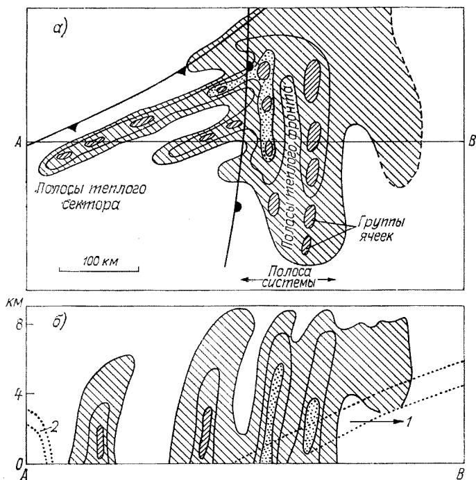
Черт. 5.2. Типизированное изображение зон радиоэха синоптического масштаба в окклюдированном циклоне и связанных с осадками систем теплого и холодного фронтов.
