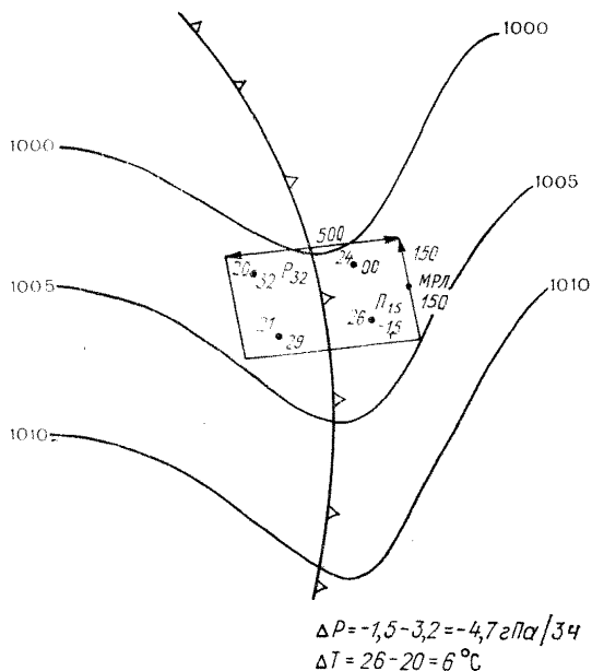
Черт. 5.14. Пример определения разности тенденций давления для уточненного синоптико-радиолокационного варианта метода прогноза шквалов.
