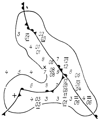
Черт. 5.9. Радиоэхо облачности и осадков за 03 ч 19 июля 1980 г. Район Актюбинска.
