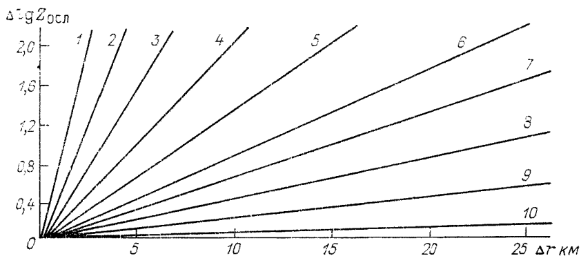
Черт. 1.16. График для расчета поправок отражаемости (\Delta \lg Z)_{\text{осл}} в зависимости от интенсивности экранирующих осадков I (мм/ч) и протяженности зоны осадков \Delta r (км).
