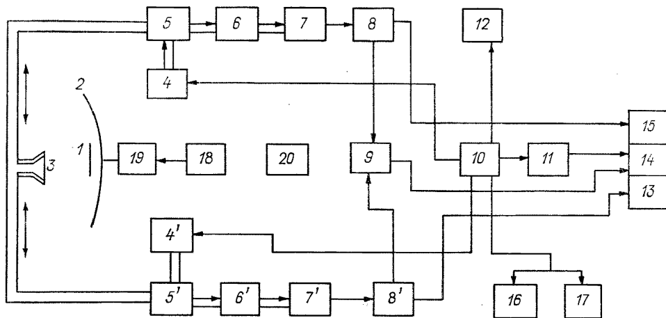
Черт. 6.8. Структурная схема радиолокатора МРЛ-5.
