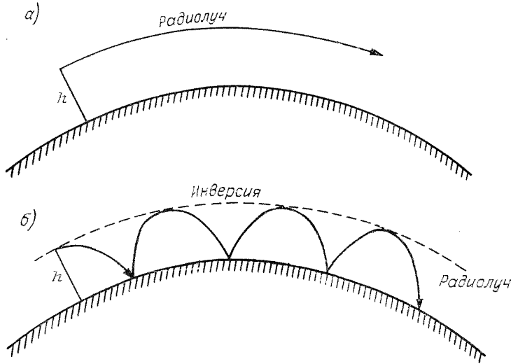
Черт. 1.8. Радиолуч над поверхностью Земли.
