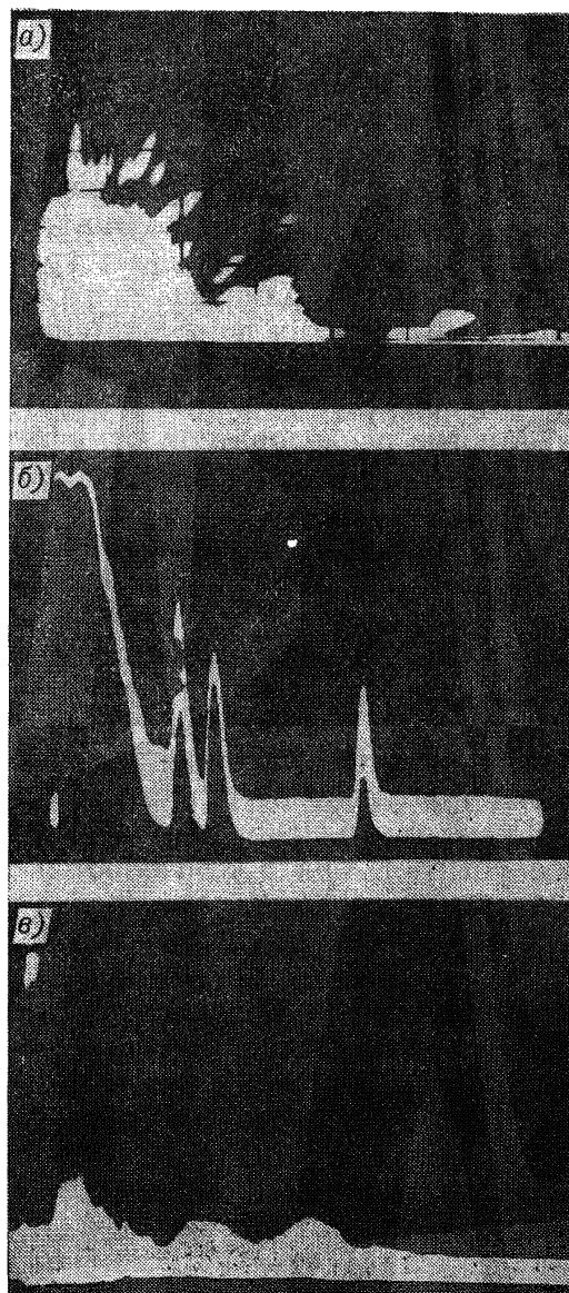
Черт. 2.21. Дискретно-когерентное радиоэхо.
