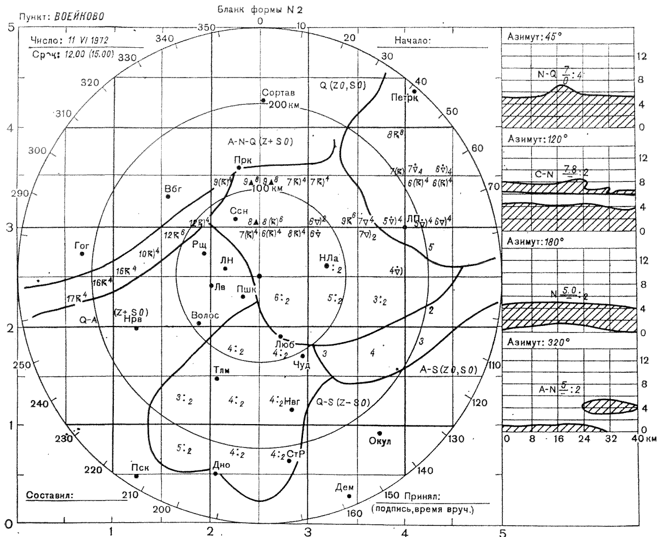
Черт. 9.2. Пример проанализированной радиолокационной информации, полученной с методиче-скими и техническими ошибками.
