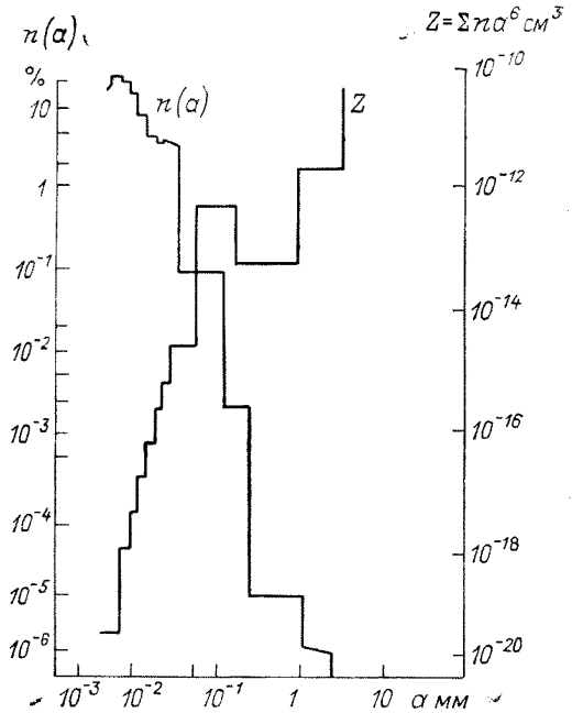
Черт. 1.13. Распределение отражаемости Z и размеров капель в облаках и осадках.
