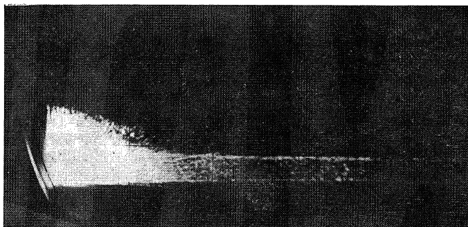
Черт. 2.13. „Яркая полоса“ при вертикальном разрезе.
