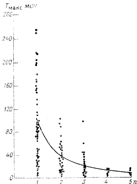
Черт. 2.7. Осредненная зависимость между временем существования очага T_{\text{макс}} и степенью его раздробленности.
