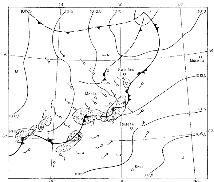
Черт. 5.1. Схематическое изображение малоподвижного холодного фронта с волнами и данными МРЛ (зоны, обозначенные точками) по кольцовке БТГМЦ (М 1:2 500 000) за 06 (09) ч 8 мая 1972 г.
