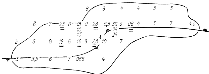
Черт. 5.6. Волна на холодном фронте. Район Алма-Аты.
