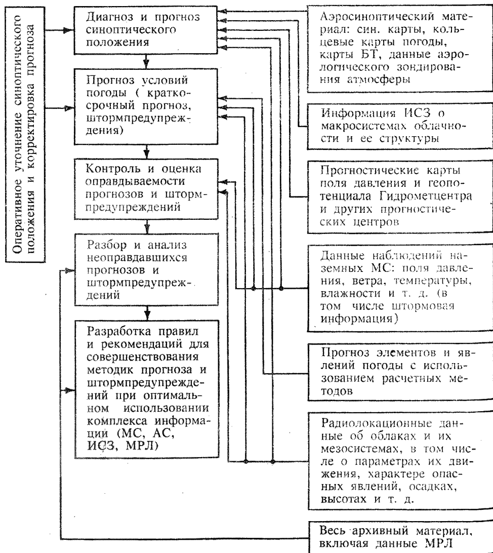
Черт. 5.12. Схема использования наземной, спутниковой и радиолокационной информации в синоптическом анализе при разработке и контроле оправдываемости прогнозов погоды.
