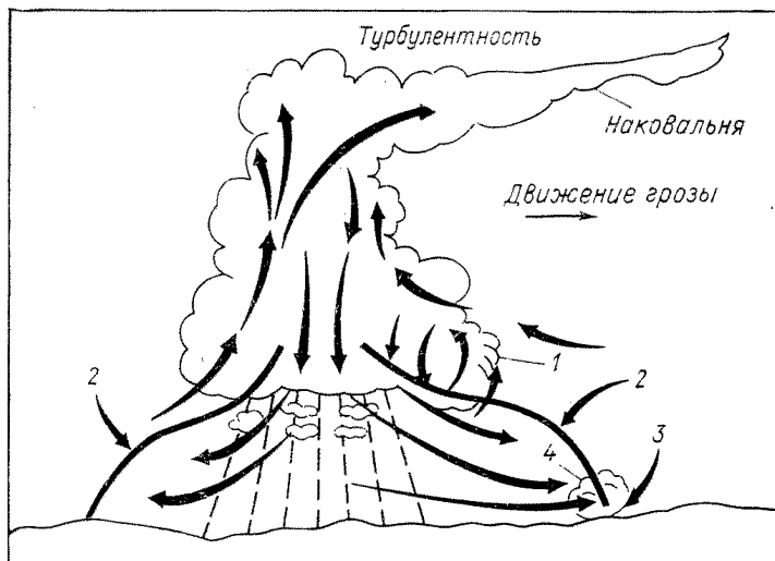
Черт. 2.1. Грозовое кучево-дождевое облаков в стадии развития с сопровождающими его опасными явлениями. 1 — шкваловый вентиль; 2 — турбулентность сдвига ветра; 3 — порыв ветра; 4 — пыль.
