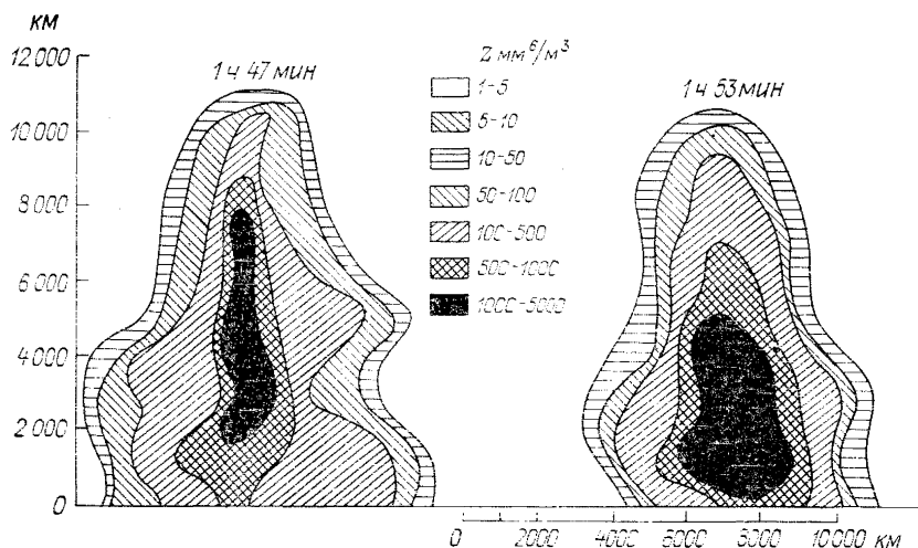
Черт. 2.8. Изменение отражаемости во времени в грозном облаке по данным за 17 августа 1954 г. (по данным Е. М. Сальмана).
