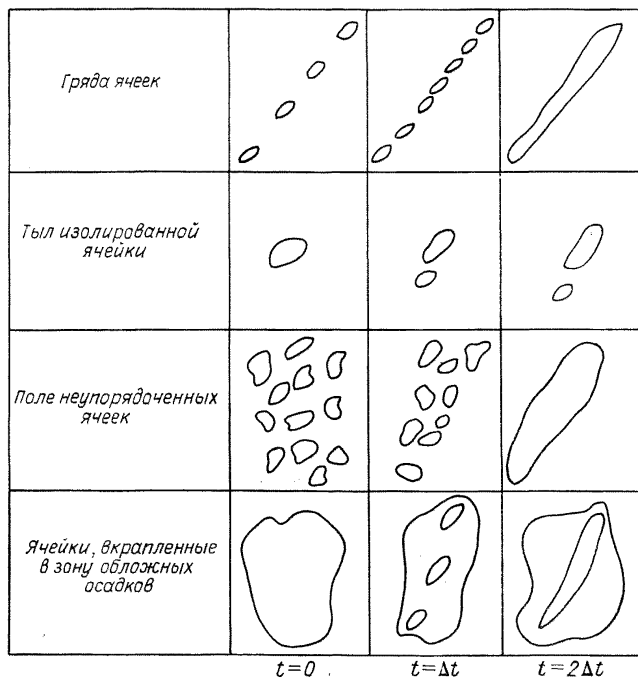
Черт. 2.12. Классификация процесса формирования линии шквалов.
