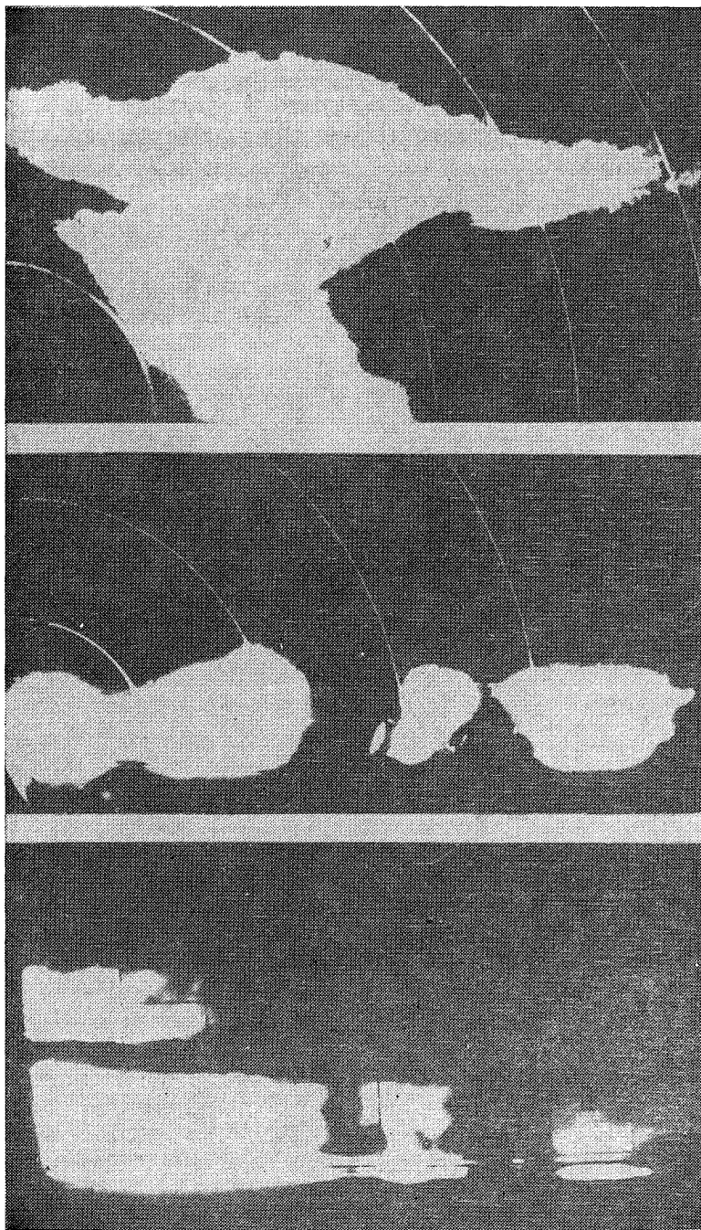
Черт. 2.14. Типичные картины радиоэха различных форм облаков в летний период года (верхние фото) и зимний период (нижнее фото).
