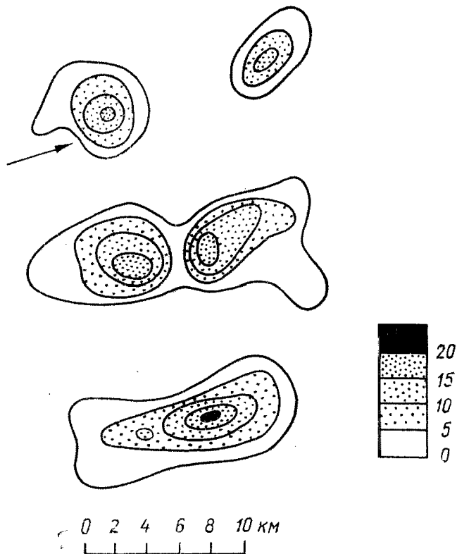
Черт. 2.2. Слияние радиоэха двух ячеек.
