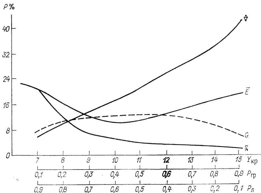
Черт. 2.19. Зависимости средних ошибок распознавания P (%) гроз ( K ), ливней ( V ) и суммарной ошибки распознавания для критерия грозоопасности Y_{кр} ( E ) и единой обучающей выборки ( G ) от априорной вероятности появления гроз P_{гр} и ливней P_{л} .
