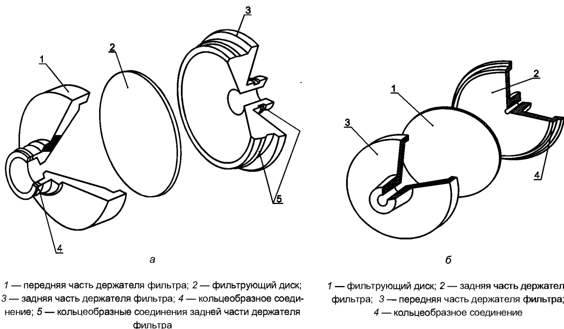
Рисунок 4 — Схема ловушки для дыма с фильтрующим диском из стекловолокна
