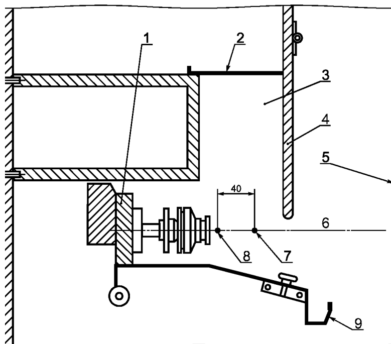
Рисунок А.2 — Шкаф ротационной курительной машины с колпаком
