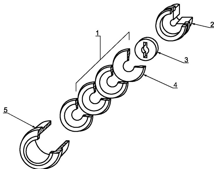
Рисунок 1 — Лабиринтовое уплотнение и перфорированный диск держателя сигарет
