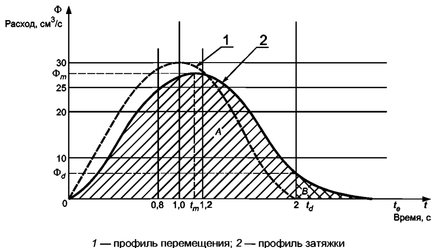
Рисунок В.1 — Схематическое изображение профиля затяжки сигареты
