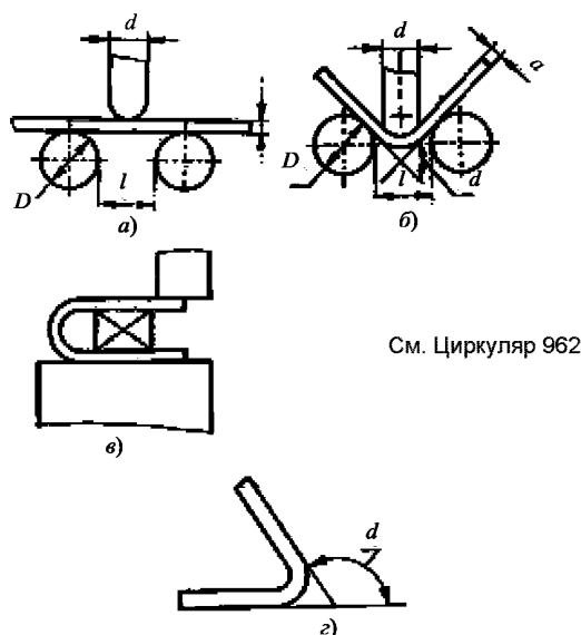
Рис. 3 Схема испытаний на изгиб
