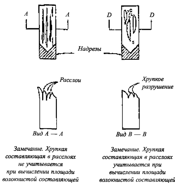
Рис. 1.3-2 Порядок учета площади кристаллических пятен в изломе
