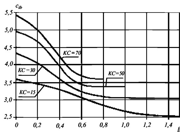
Рис. 9-2 Коэффициент c_{tb} в зависимости от коэффициента \beta
