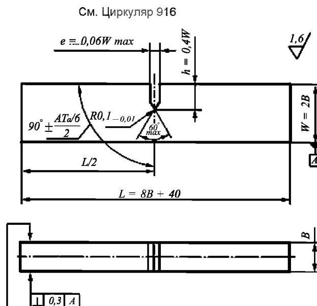
Рис. 2-2 Предпочтительный тип образцов для испытаний на СТОД
