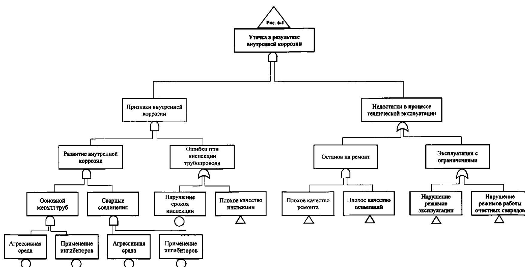
Рис. 6-3 Дерево отказов для аварии, связанной с внутренней коррозией подводного трубопровода
