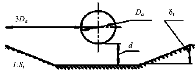
Рис. 2.3 Расположение трубопровода в траншее
