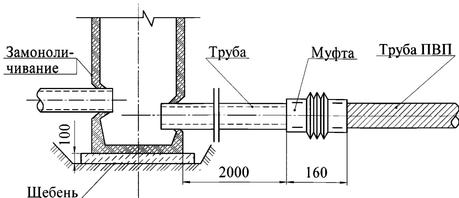
Рисунок 7 – Схема соединения колодца с дренажной трубой
