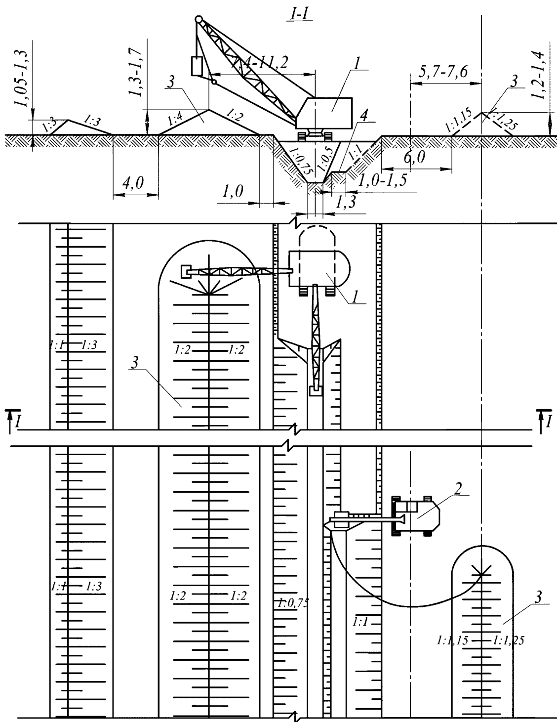
1 – экскаватор-драглайн; 2 – экскаватор с обратной лопатой; 3 – отвал грунта;
