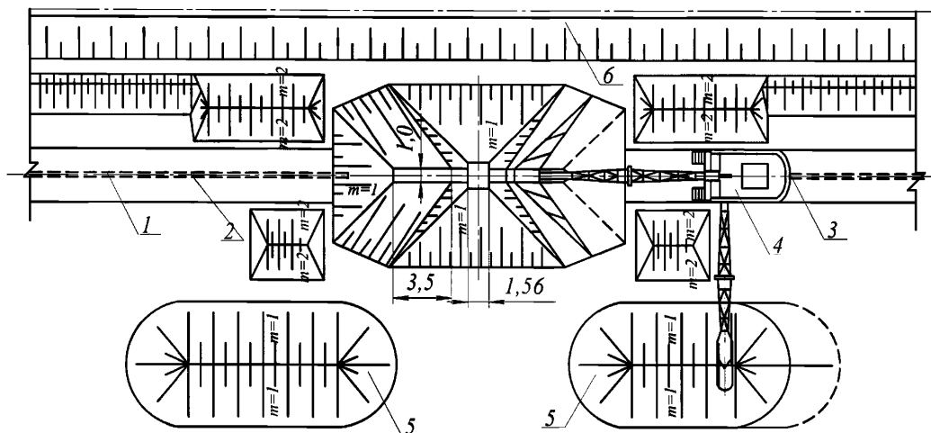
1 – дренажная линия; 2 – ось первой проходки экскаватора; 3 – ось второго прохода экскаватора; 4 – экскаватор; 5 – отвалы минерального грунта; 6 – осушительная траншея
