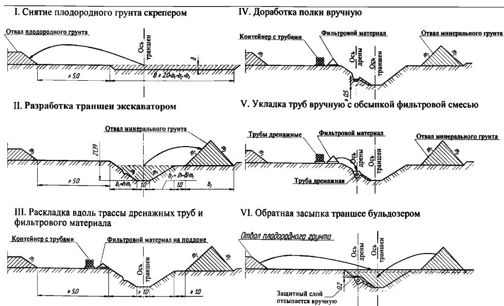
Рисунок 3 – Технологическая схема строительства закрытых дрен широкотраншейным способом
