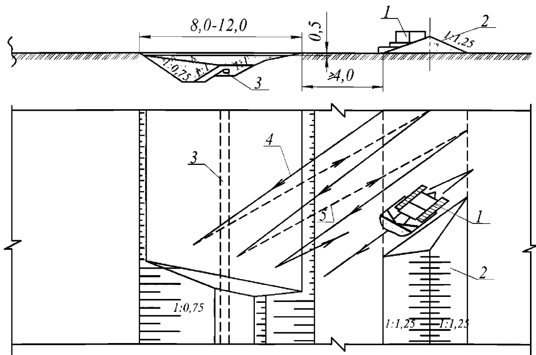
Рисунок В.4.2 – Обратная засыпка водоотводящей части траншеи
