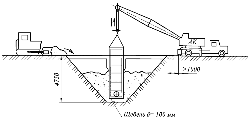
Рисунок 6 – Схема монтажа колодцев по трассе дрены
