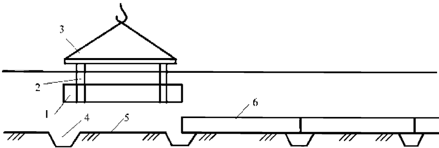
Рисунок 2 – Схема укладки трубопровода по циклической технологии (укладка звеньев)
