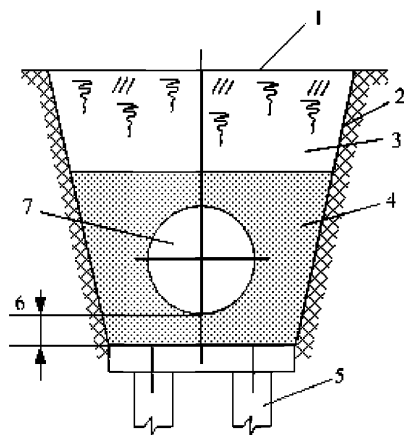
Рисунок 4 – Расположение трубопровода в траншее с укреплением дна железобетонной плитой
