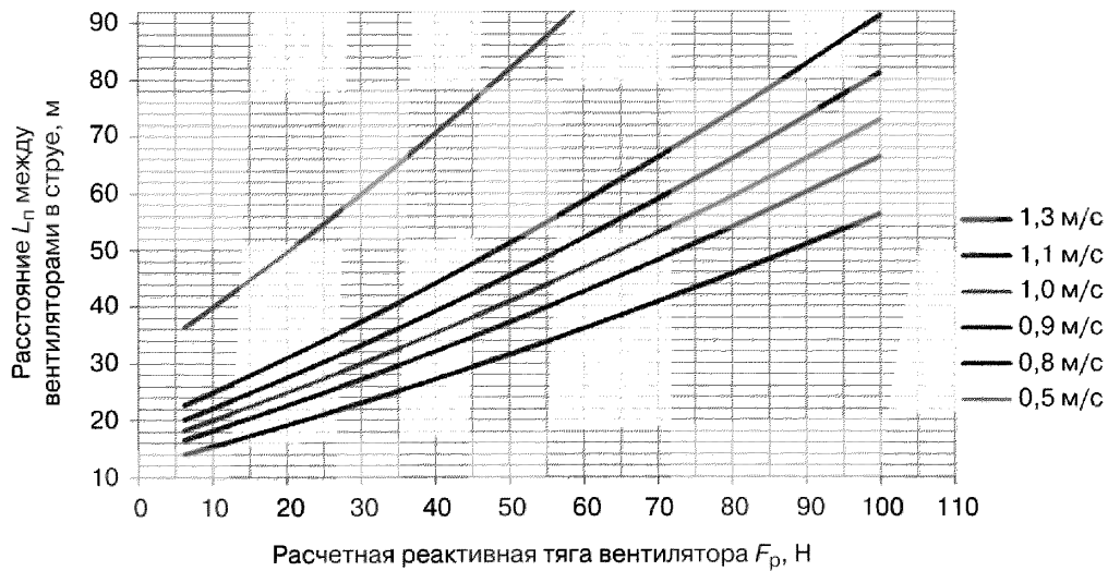
Рисунок 6.9 – График зависимости продольного расстояния между вентиляторами L_{\text{п}} (в струе) от расчетной реактивной тяги F_p вентилятора при различных значениях v_{x \min}
