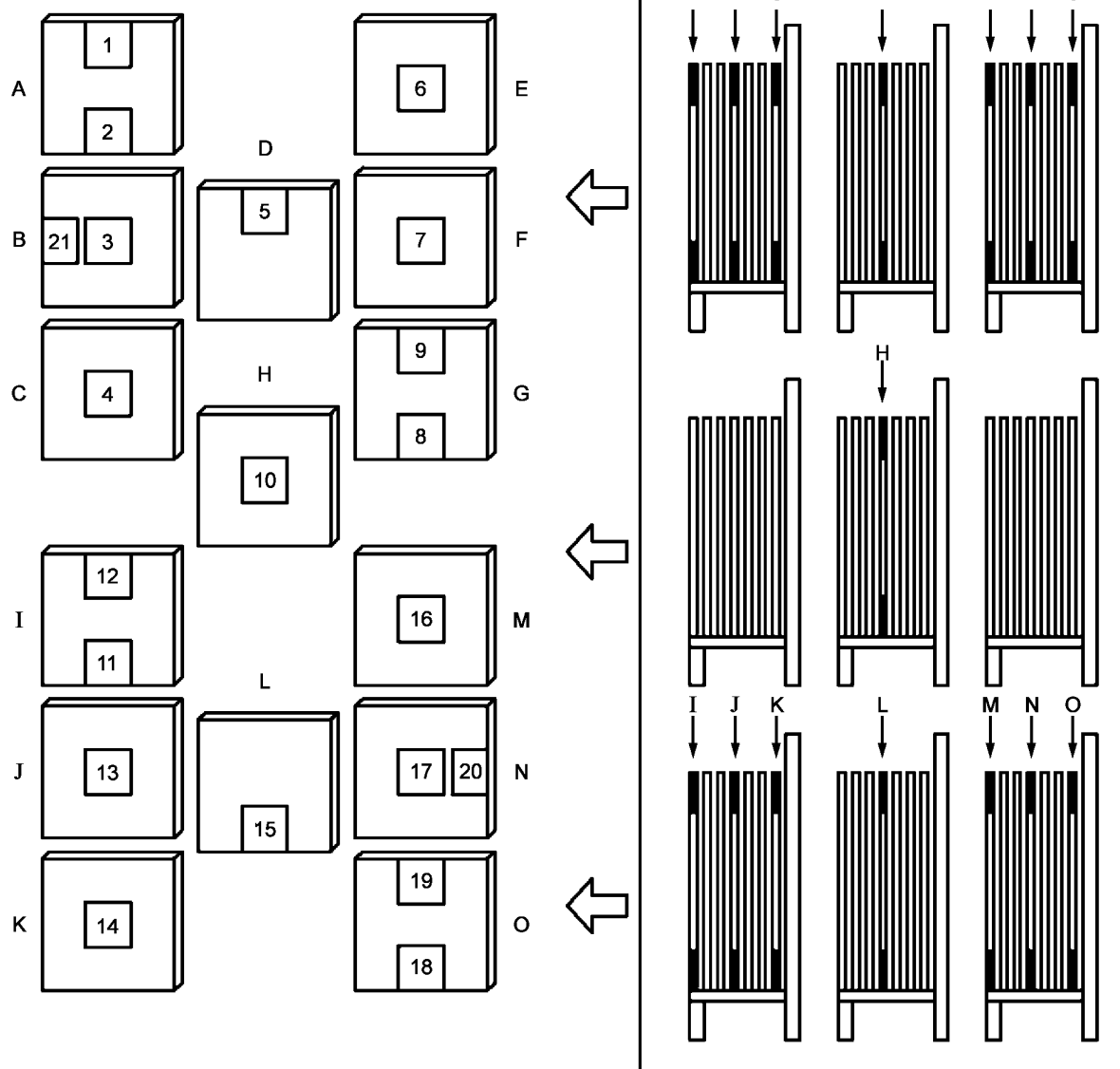
Рисунок А.8 — Третья категория — 6 или 8, или 9... стеллажей — полная загрузка
