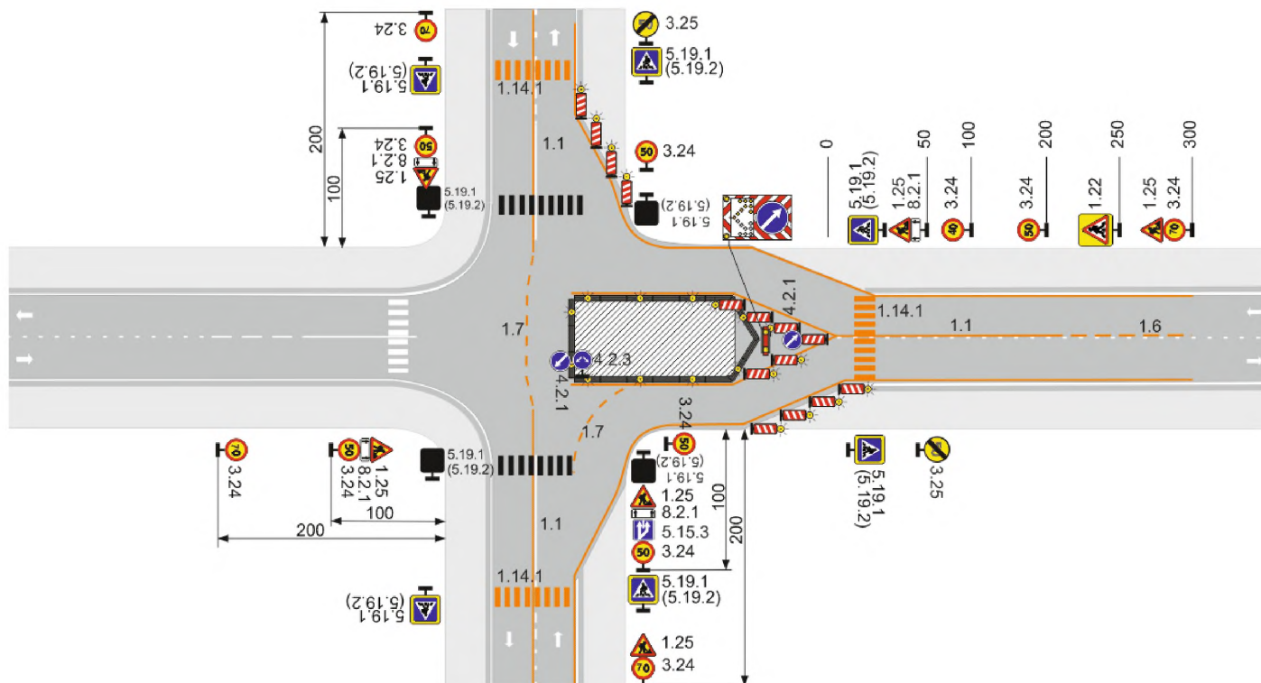
Рисунок Б.11 – Двухполосная дорога. Рабочая зона производства долговременных работ на пересечении в одном уровне на всей ширине проезжей части. Пропуск транспортных средств по обочинам
