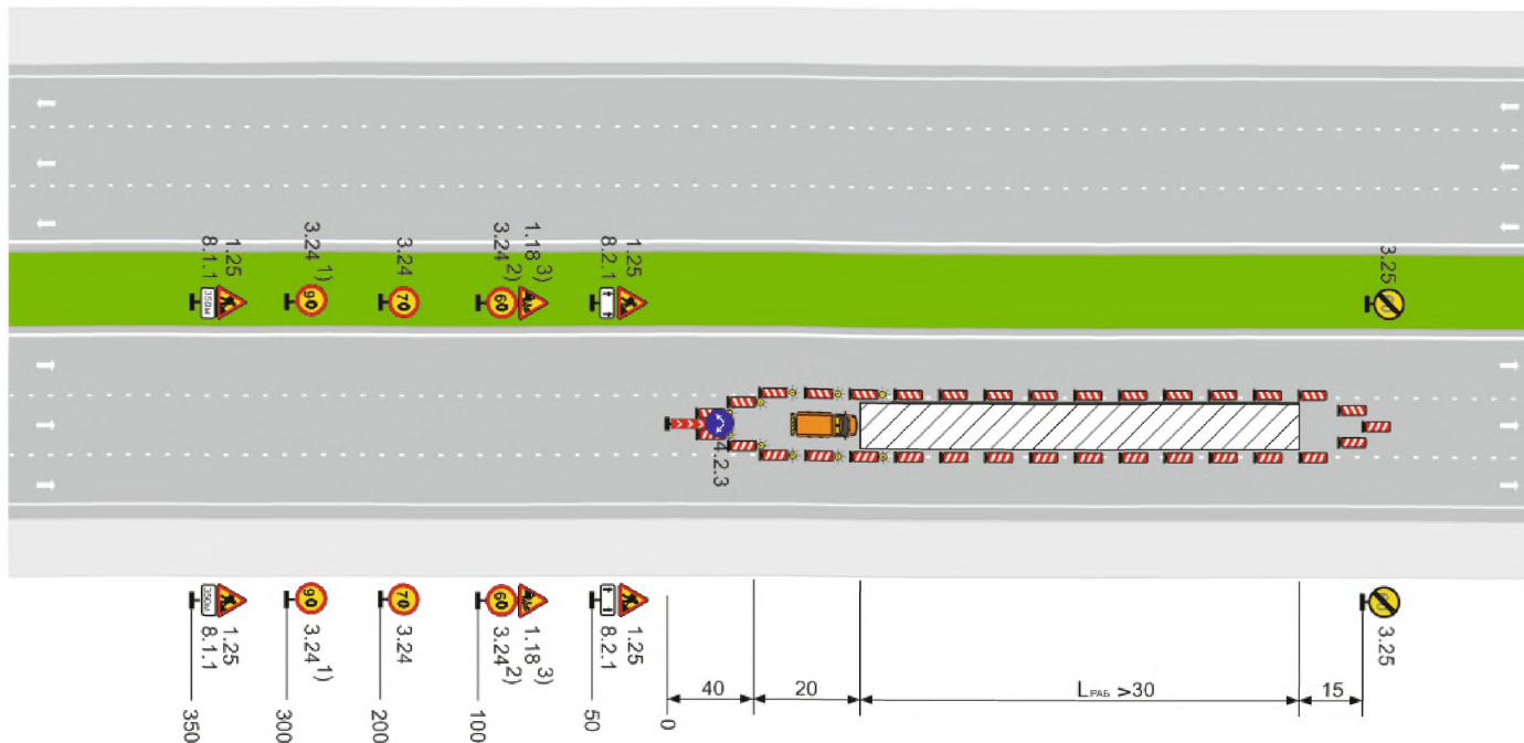
Рисунок Б.40 – Автомагистраль, скоростная дорога, многополосная дорога обычного типа с разделительной полосой. Рабочая зона производства краткосрочных работ на средней полосе (полосах). Пропуск транспортных средств по существующим свободным полосам
