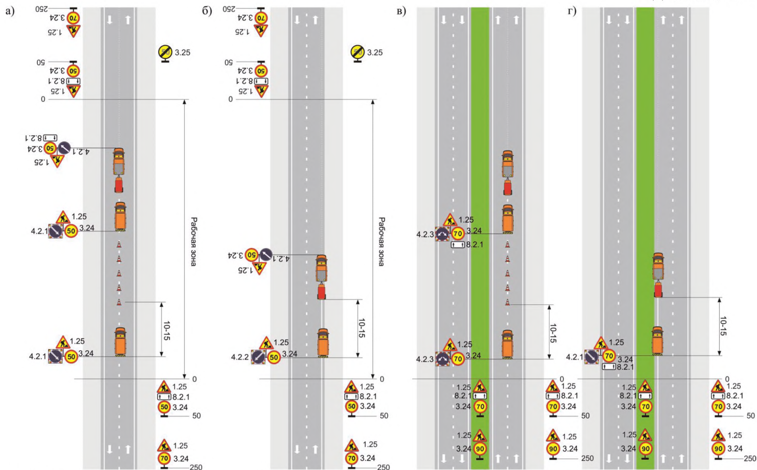
Рисунок Б.38 – Автомагистраль, скоростная дорога, многополосная дорога обычного типа. Производство краткосрочных передвижных работ по нанесению дорожной разметки осевых линии (а), линии границ полос движения (б), крайевых линии обочины (в), крайевых линии разделительной полосы (г)
