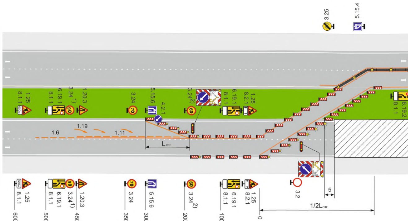
Рисунок Б.28 – Автомагистраль, многополосная дорога обычного типа с разделительной полосой. Рабочая зона производства долговременных работ на всей ширине проезжей части. Пропуск транспортных средств по полосе встречного движения с переводом через разделительную полосу
