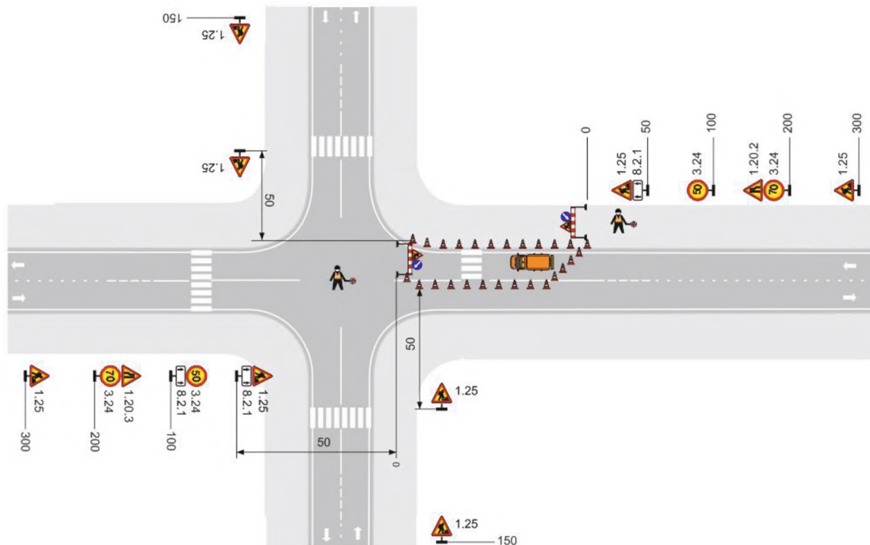
Рисунок Б.39 – Пересечение автомобильных дорог в одном уровне. Рабочая зона производства краткосрочных работ по нанесению дорожной разметки на полосе движения. Пропуск транспортных средств по полосе встречного движения с помощью регулировщиков (при необходимости допускается увеличивать количество регулировщиков)
