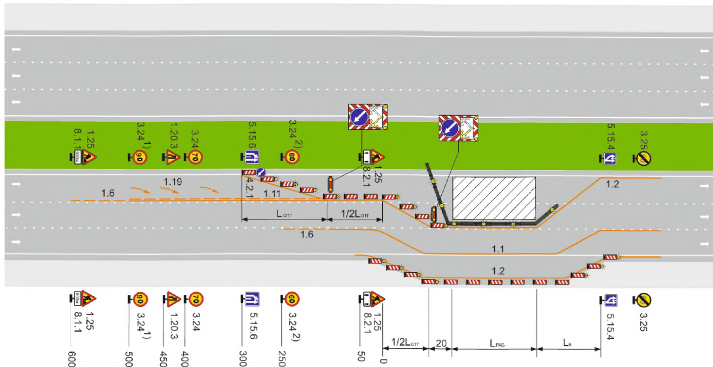
Рисунок Б.23 – Автомагистраль, скоростная дорога, шестиполосная дорога обычного типа. Рабочая зона производства долговременных работ на крайней левой и средней полосах движения. Пропуск транспортных средств по одной полосе и обочине
