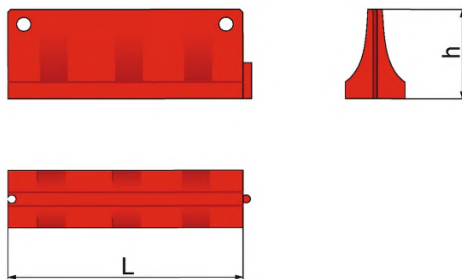
Рисунок 6 – Защитный блок из полимерного материала
