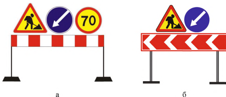
Рисунок 11 – Комплекс дорожных знаков переносной (а, б)
