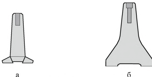
а – высота 50 и 65 см; б – высота 80 см Рисунок 5 – Временные защитные барьеры
