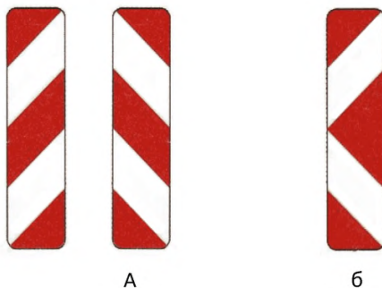
Рисунок 2 – Виды (а, б) направляющих пластин
