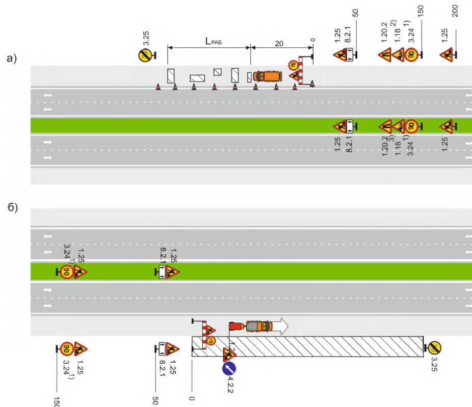
Рисунок Б.37 – Автомагистраль, скоростная дорога, многополосная дорога обычного типа. Рабочая зона производства краткосрочных работ на обочине (а) или откосе (б)
