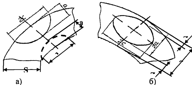
Рис. 9.2. Несплошности, ориентированные в кольцевом направлении (поперек продольной оси оборудования или трубопровода, или вдоль сварного соединения):
