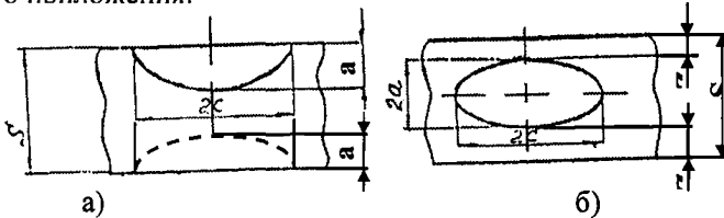
Рис. 9.1. Несплошности, ориентированные в продольном направлении (вдоль продольной оси оборудования или трубопровода, или поперек сварного соединения):
