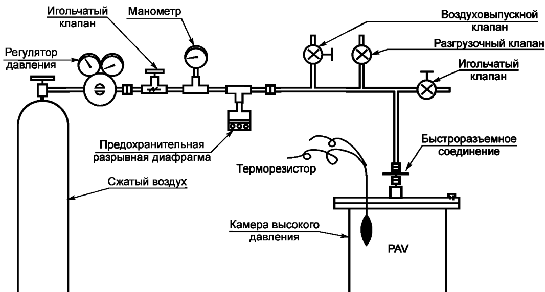
Рисунок 1 — Схема испытательного оборудования
