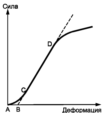
Рисунок А.1 — График зависимости силы от деформации
