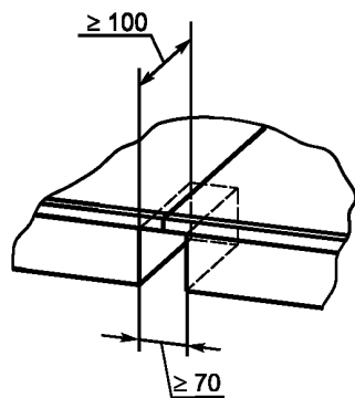
Рисунок 4 — Свободное пространство для крепления комплекта сетки
